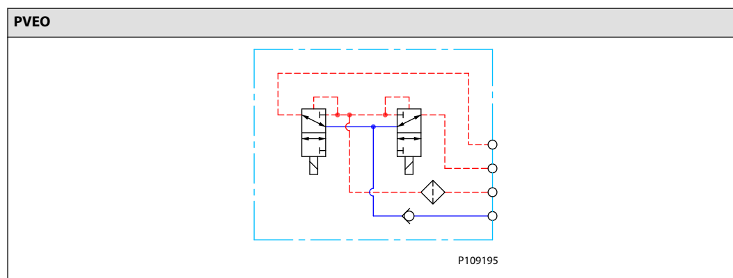
PVEO 原理图
