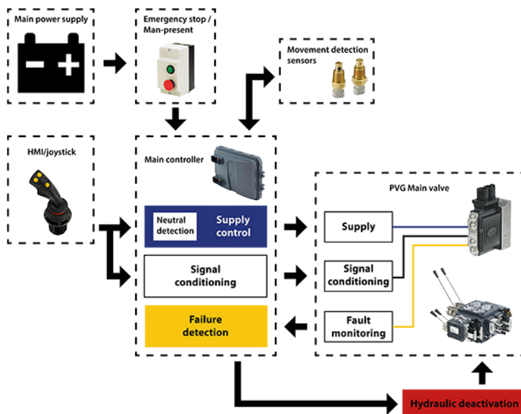
电路框图
