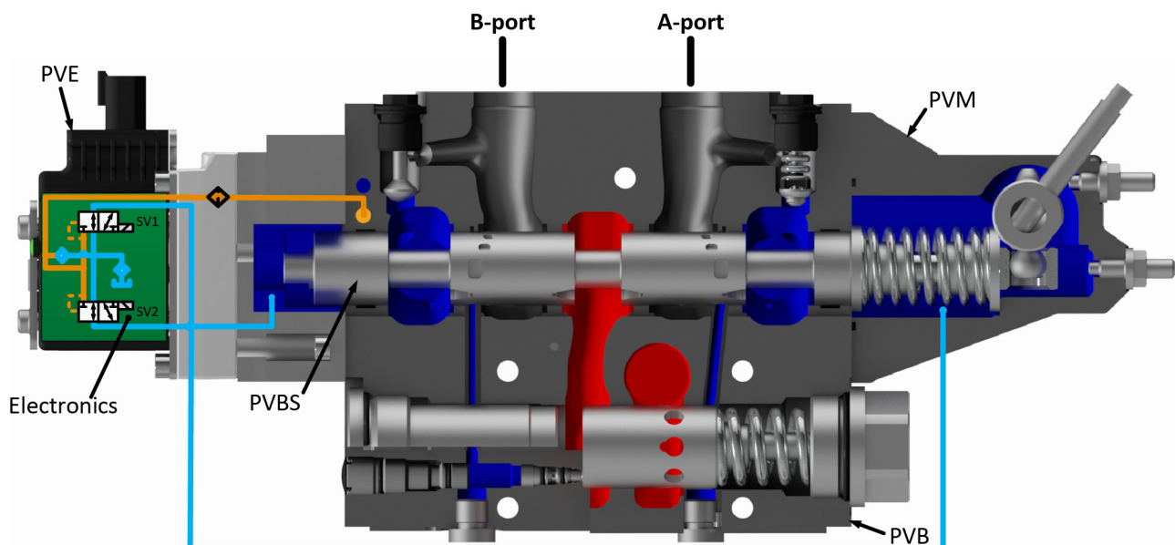
PVG 256 带 PVEO
