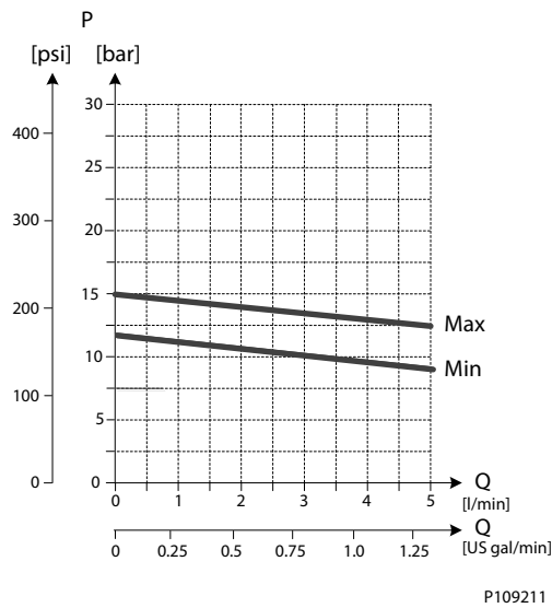
先导减压阀性能
