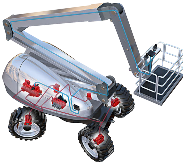
高空作业平台
