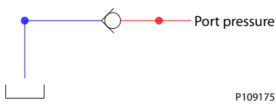
PVLA 原理图
