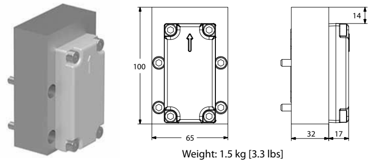
PVMD 尺寸
