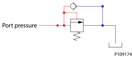
PVLA 原理图
