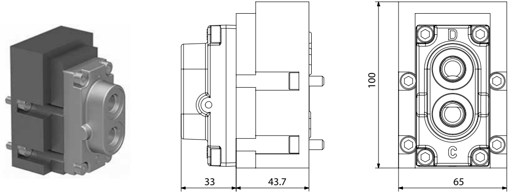
PVH 尺寸
