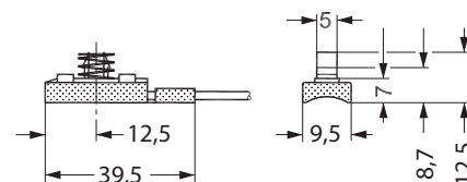
Oberflächentemperatur-Sensor
