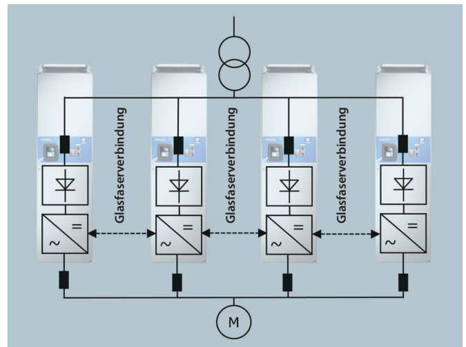
Beispiel einer VACON DriveSynch-Konfiguration.
