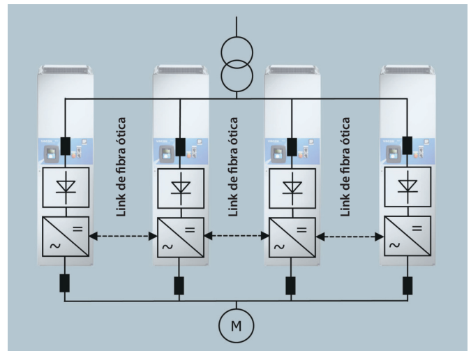
Exemplo de configuração VACON® DriveSynch.
