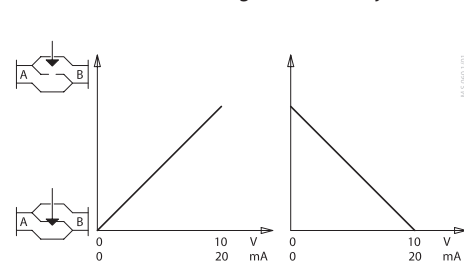
BV:2/32786 Directe of omgekeerde bedrijfsmodus
