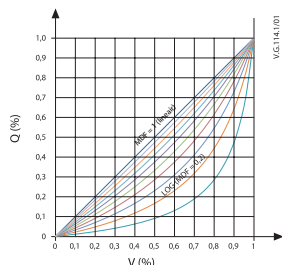
Alfawaardecurve AV:4/32772
