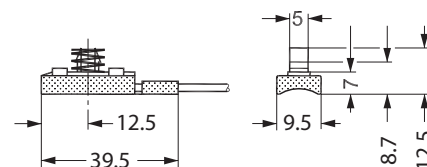
Oppervlaktetemperatuursensor
