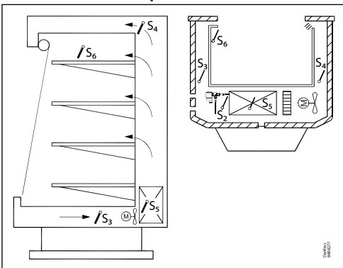
Figura 13: Esempi di configurazioni della vetrina con due sezioni di refrigerazione controllate da una valvola AKV (solo versione a bobina singola)
