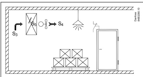
Figura 14: Configurazione della cella frigorifera con funzione di controllo porta, luce e calore
