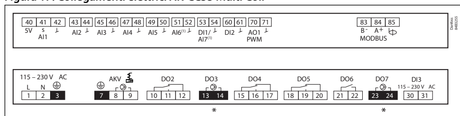
Figura 17: Collegamenti elettrici AK-CC55 Multi Coil
