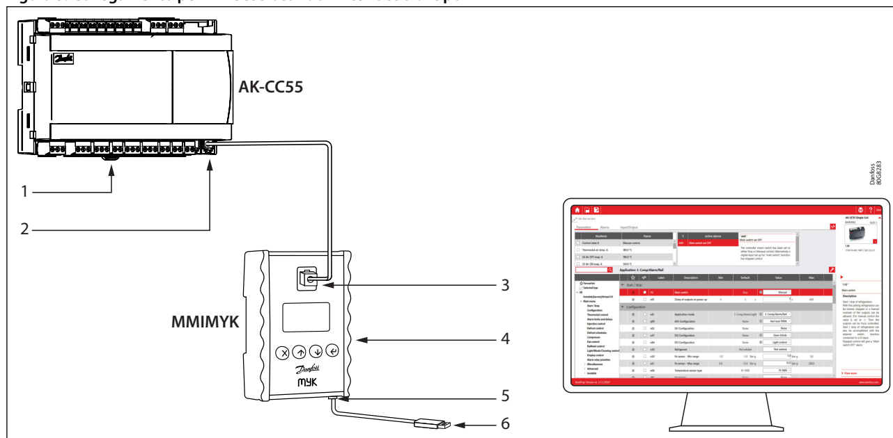
Figura 5: Collegamento per AK-CC55 usando l'interfaccia di tipo MMIMYK
