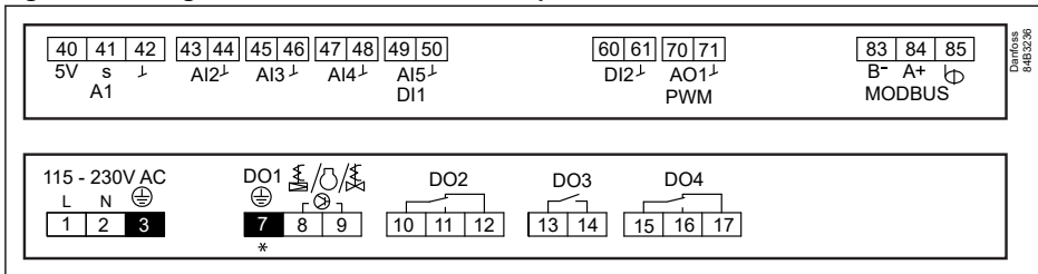
Figura 15: Collegamenti elettrici AK-CC55 Compact
