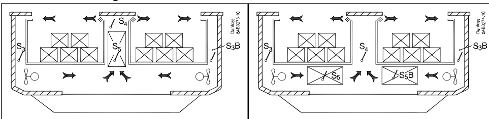
Figura 14: Configurazione della cella frigorifera con funzione di controllo porta, luce e calore
