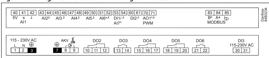
Figura 16: Collegamenti elettrici bobina singola AK-CC55
