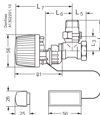
Кутовий клапан з термостатичним елементом RA 2992
