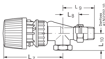
Осьовий клапан з термостатичним елементом RA 2991
