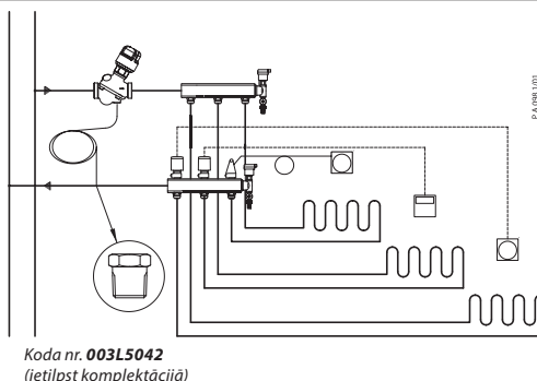
3. att.) AB-PM grīdas apsildes sistēmas sazarotajā cauruļvadā
