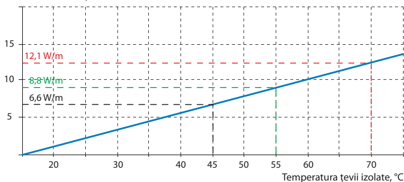
Fig. 1 – Pierderea de căldură a țevelor izolate.
