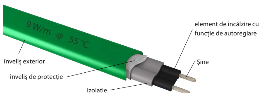
Fig. 3 - Construcția cablului SLC
