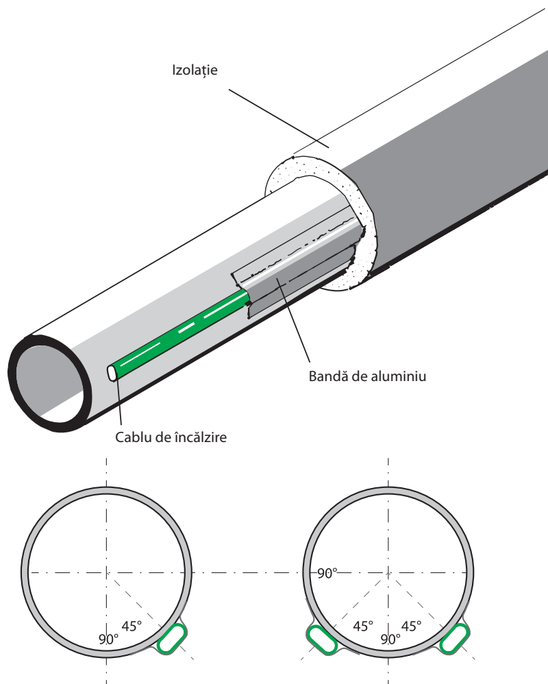
Modul în care se recomandă instalarea liniilor de cablu pe conductă
