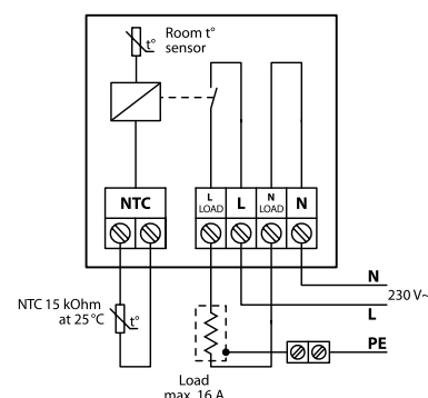
Schemat DEVireg™ Smart
