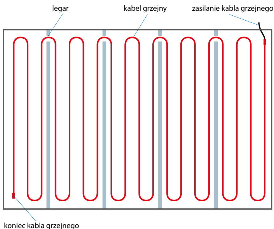
Montaż ogrzewania podłogi drewnianej na legarach
