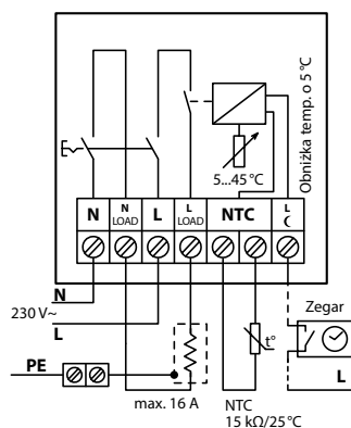
Schemat DEVIreg™ 530
