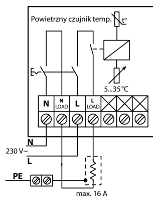
Schemat DEVIreg™ 531
