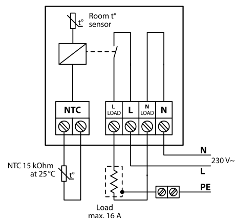
Schemat DEVireg™ Tocht
