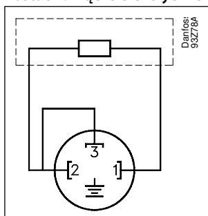
Postać 1: Złącze elektryczne
