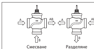
Фиг. 1: Съединение за смесване или разделяне
