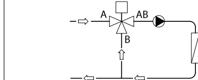
Фиг. 2: Смесителен клапан, използван в приложение за смесване
