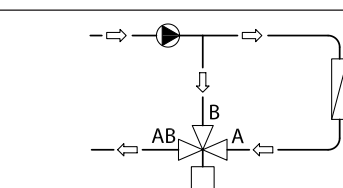
Фиг. 3: Смесителен клапан, използван в приложение за разделяне
