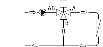
Фиг. 4: Разделителен клапан, използван в приложение за разделяне
