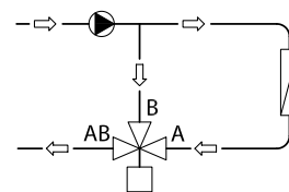
Fig. 3: válvula mezcladora en una aplicación de desvío
