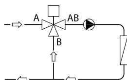
Fig. 2: válvula mezcladora en una aplicación de mezcla
