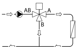
Fig. 4: válvula diversora en una aplicación de desvío
