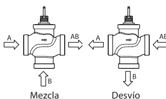
Fig. 1: conexión de mezcla o desvío
