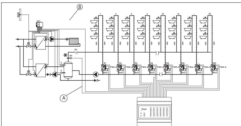
Figur 11 – installationsschema för desinficering och temperaturregistrering
