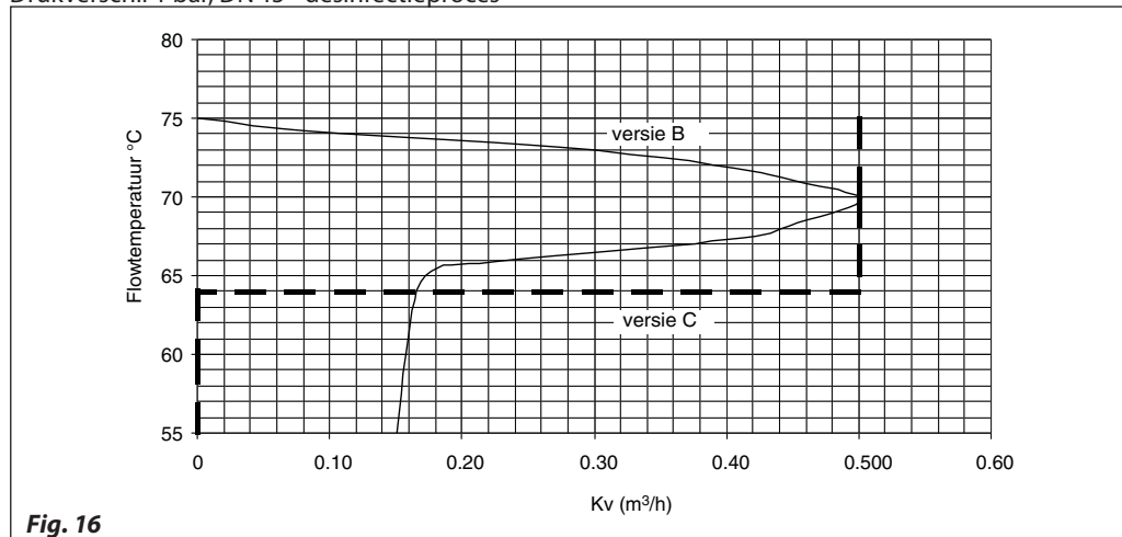
Drukverschil 1 bar, DN 15 - desinfectieproces
