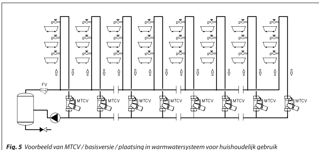
Fig. 5 Voorbeeld van MTCV / basisversie / plaatsing in warmwatersysteem voor huishoudelijk gebruik
