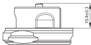
Sluitingspunt (maat) voor DN 10-32
