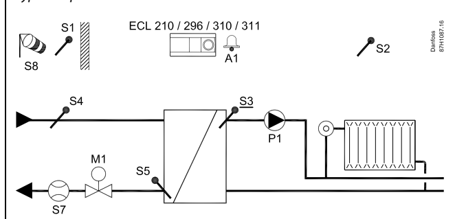
Typická aplikace A230.1:
