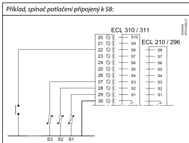
Příklad, relé potlačení připojené k S8:
