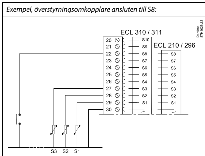
Exempel, överstyrningsrelä anslutet till S8:
