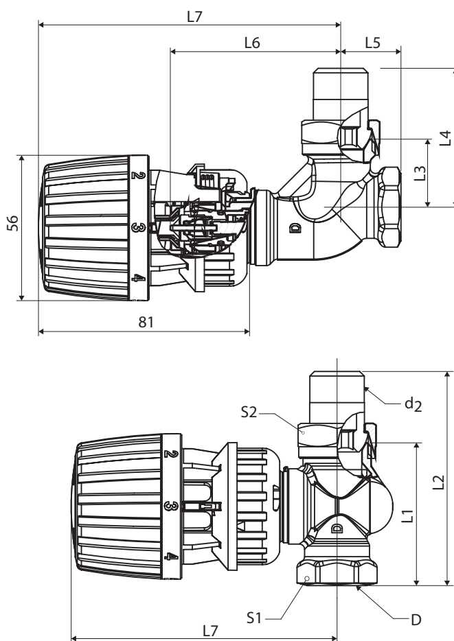
RA-DV DN 20 Durchgangs- und Eckventil/Fühler RA 2990
