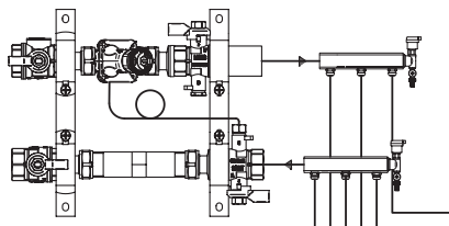
4. att.) AB-PM savienojumu komplekts sazarotajam cauruļvadam (horizontāls vai vertikāls savienojums)
