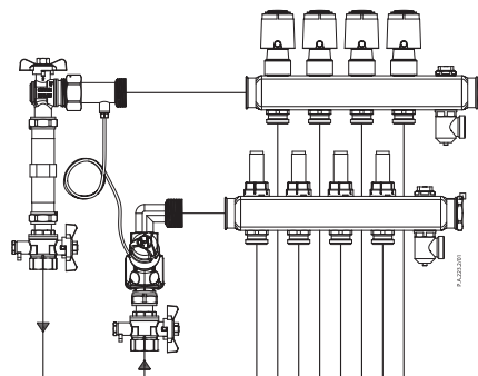
AB-PM siltuma skaitītāja savienojumu komplekts, vertikāls
