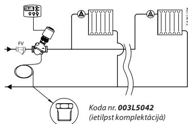
2. att.) AB-PM radiatora apsildes sistēmās
