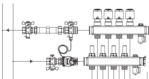
AB-PM siltuma skaitītāja savienojuma statīva komplekts
