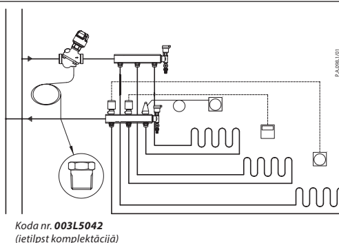
3. att.) AB-PM grīdas apsildes sistēmas sazarotajā cauruļvadā
