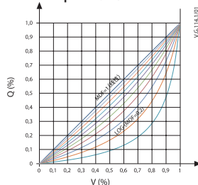
AV:4 / 32772 Alpha 值曲线
