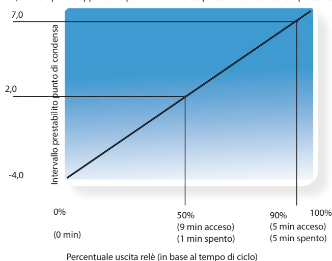
8,0 Esempio di rapporto tra punto di condensa prestabilito e uscita relè percentuale
