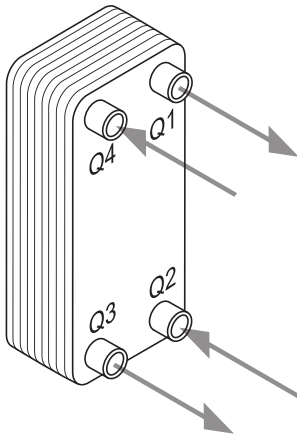
Condenser
