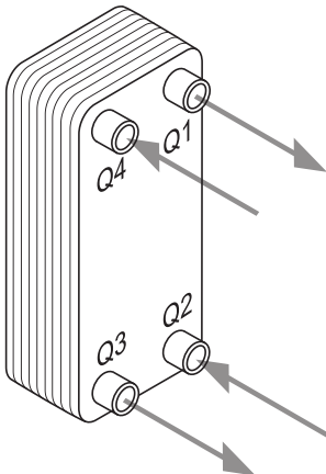
Skraplacz
