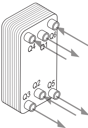
Zweikreis-Verflüssiger
