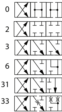
DG4V-3(S)-*B
