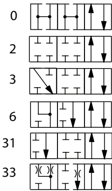
DG4V-3(S)-*BL
