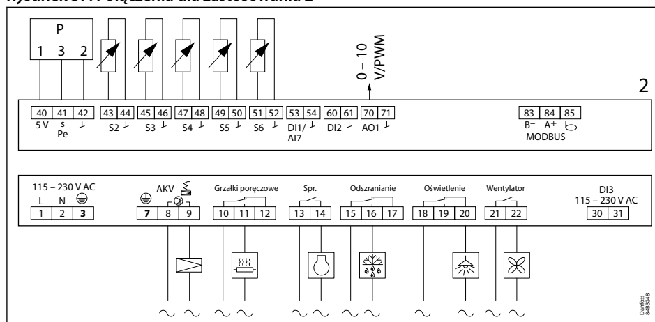
Rysunek 37: Połączenia dla zastosowania 2
