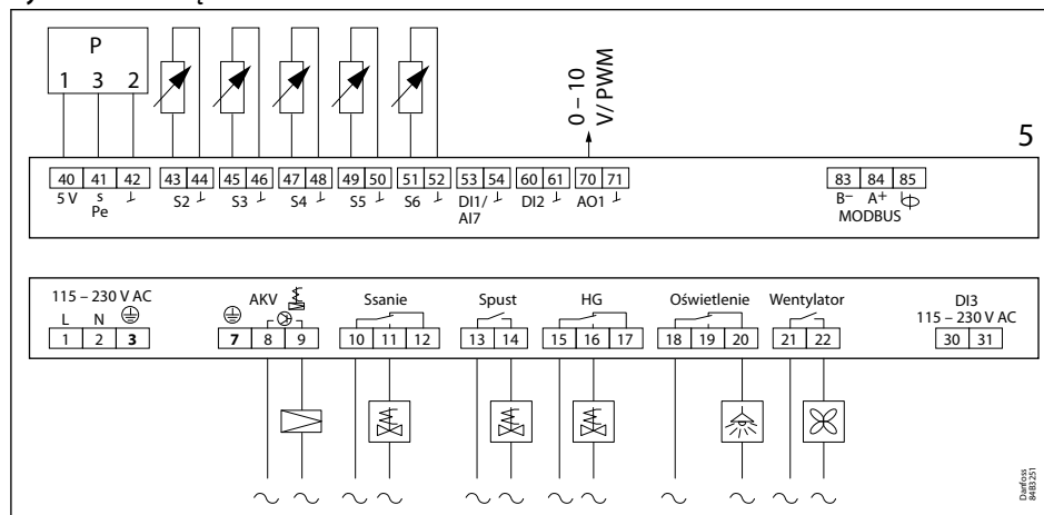
Rysunek 40: Połączenia dla zastosowania 5
