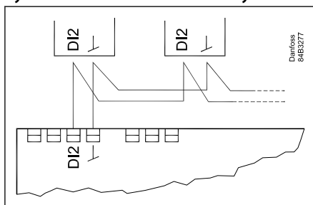
Rysunek 50: Odszranianie koordynowane poprzez połączenia kablowe
