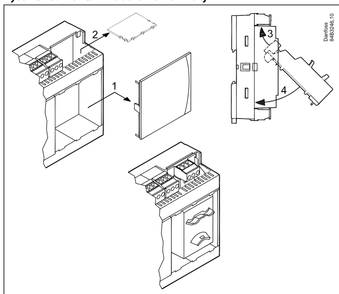
Rysunek 3: Montaż modułu komunikacji
