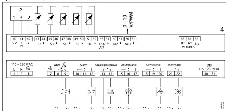
Rysunek 39: Połączenia dla zastosowania 4
