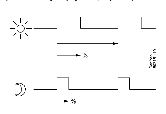
Rysunek 22: Regulacja grzałki poręczowej w zależności od obciążenia w dzień/w nocy
