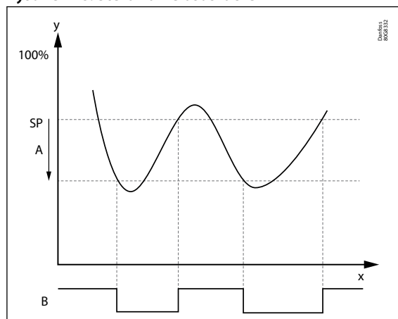
Rysunek 28: Sterowanie osuszaczem
