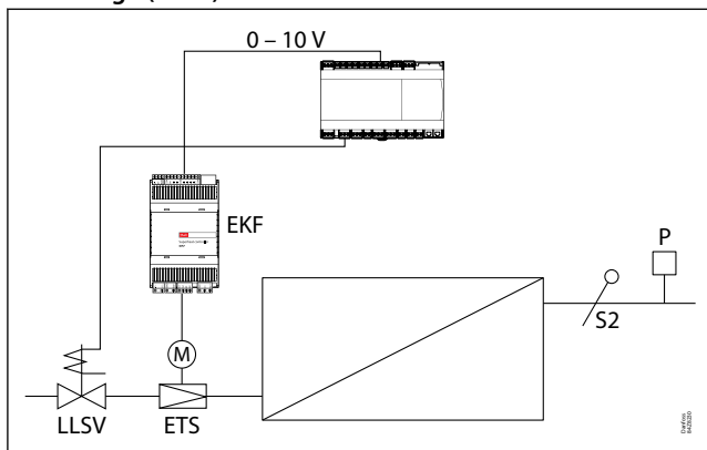
Rysunek 9: Sterowanie wtryskiem za pomocą zaworu krokowego i zaworu elektromagnetycznego rurociągu ciecowego (LLSV)
