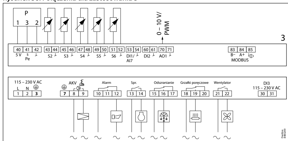
Rysunek 38: Połączenia dla zastosowania 3
