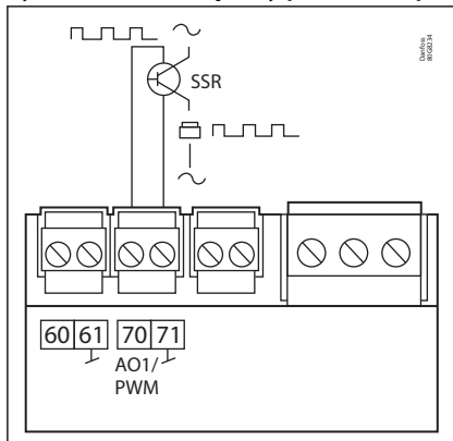
Rysunek 48: Zewnętrzny przełącznik półprzewodnikowy do grzałki poręczowej
