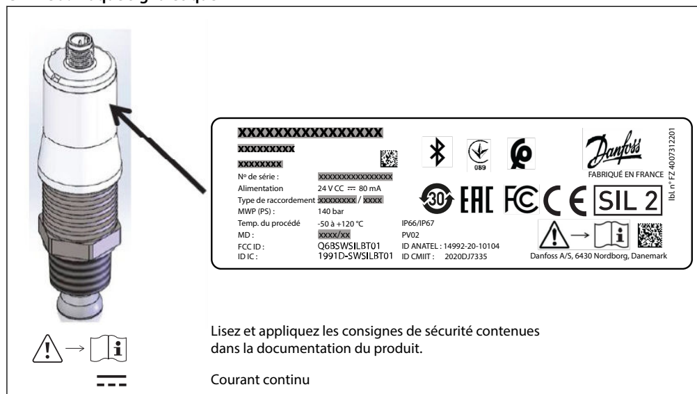
Chiffre 9: Plaque signalétique
