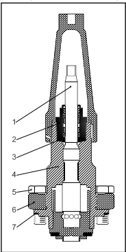
Фигура 23: Модуль запорного клапана ICFS 25
