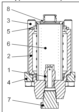
Фигура 10: Расширенный модуль сетчатого фильтра ICFF 20E
