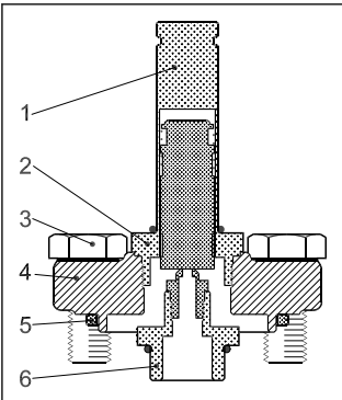
Фигура 15: Модуль электронного расширительного клапана ICFA 20
