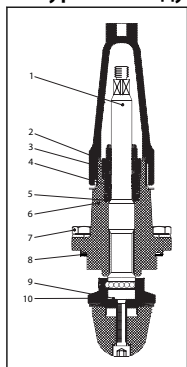
Фигура 35: Модуль ручного регулирующего клапана REG-SB 50 / REG-SB 65
