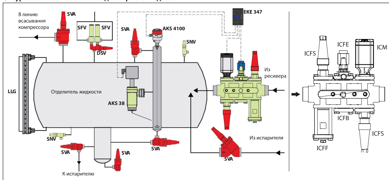
Фигура 3: Сочетание клапанов для впрыска жидкости
