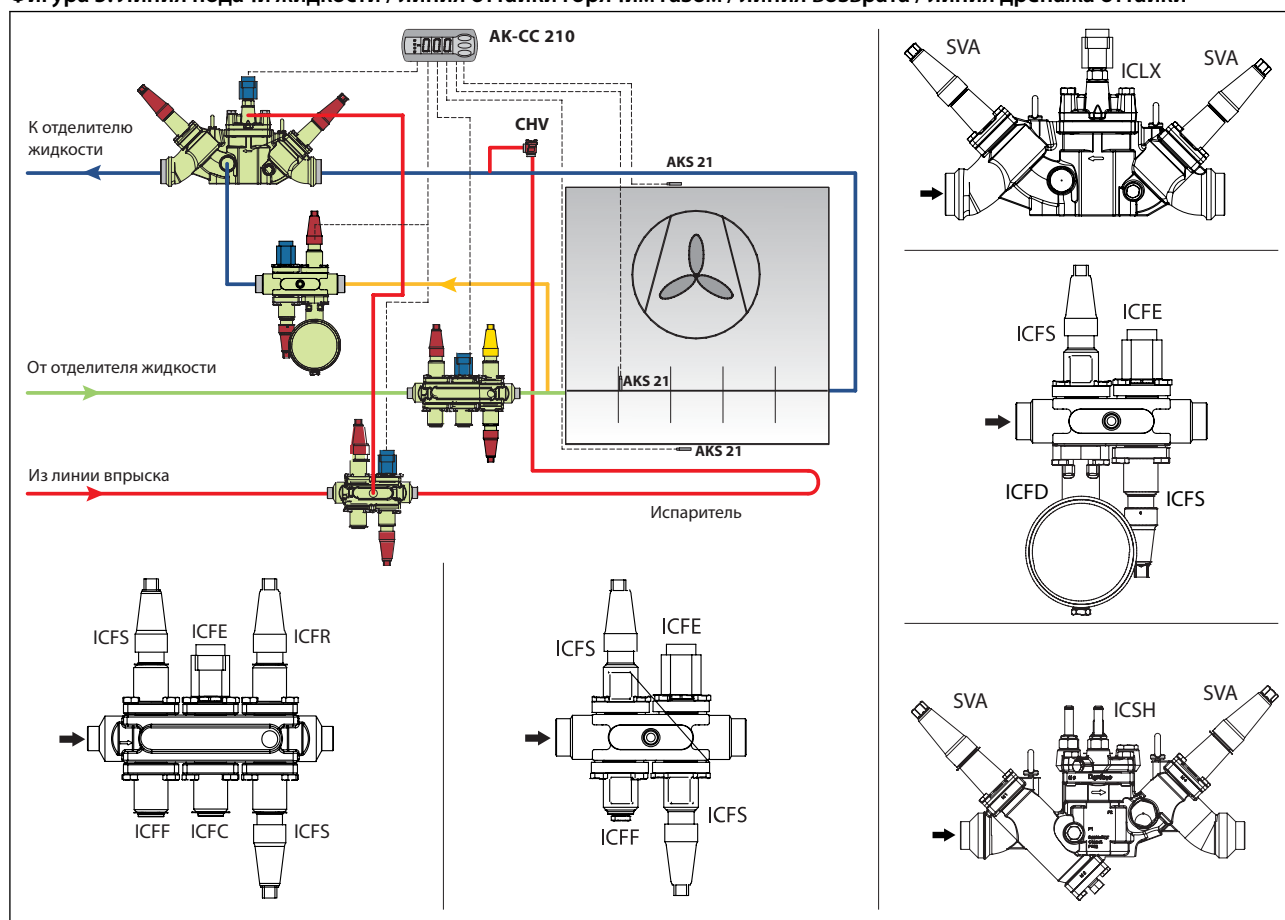
Фигура 5: Линия подачи жидкости / линия оттайки горячим газом / линия возврата / линия дренажа оттайки
