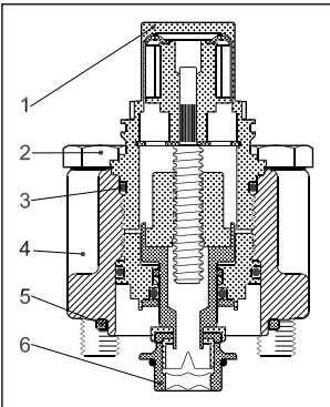
Фигура 19: Модуль электроприводного клапана ICM 20-A, 20-B или 20-C
