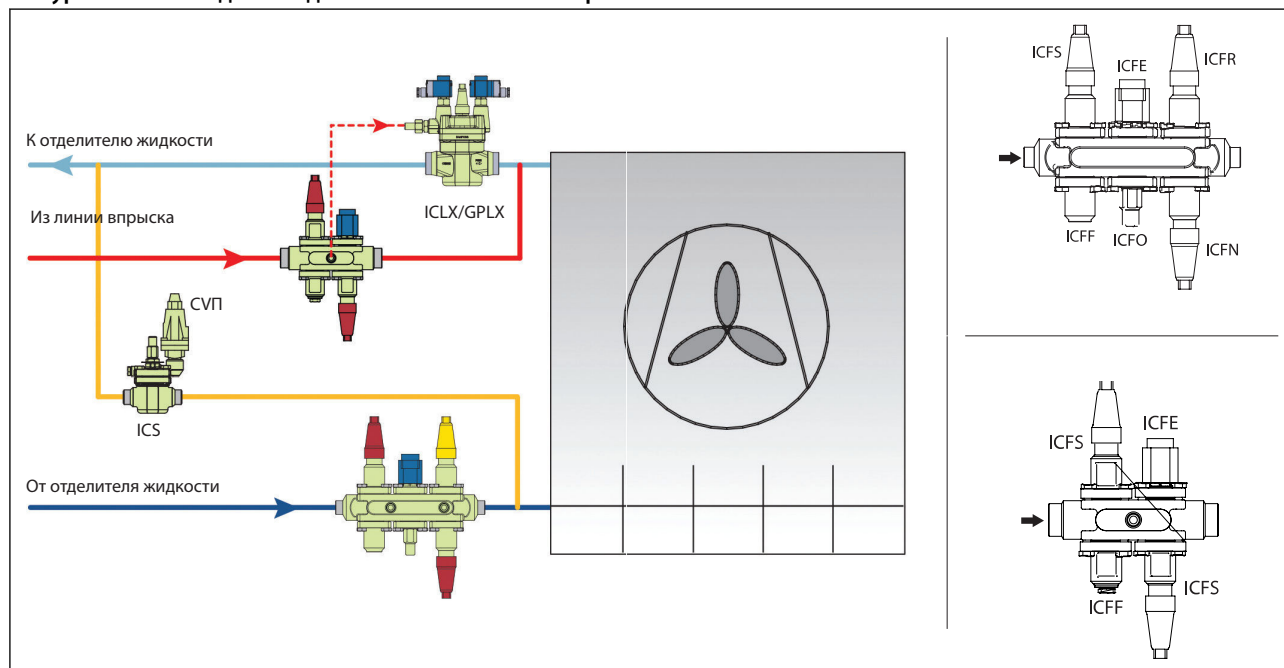
Фигура 2: Линия подачи жидкости / линия оттайки горячим газом
