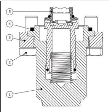
Фигура 17: Модуль обратного клапана ICFC 20P1
