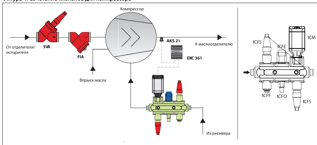
Фигура 4: Сочетание клапанов для компрессора
