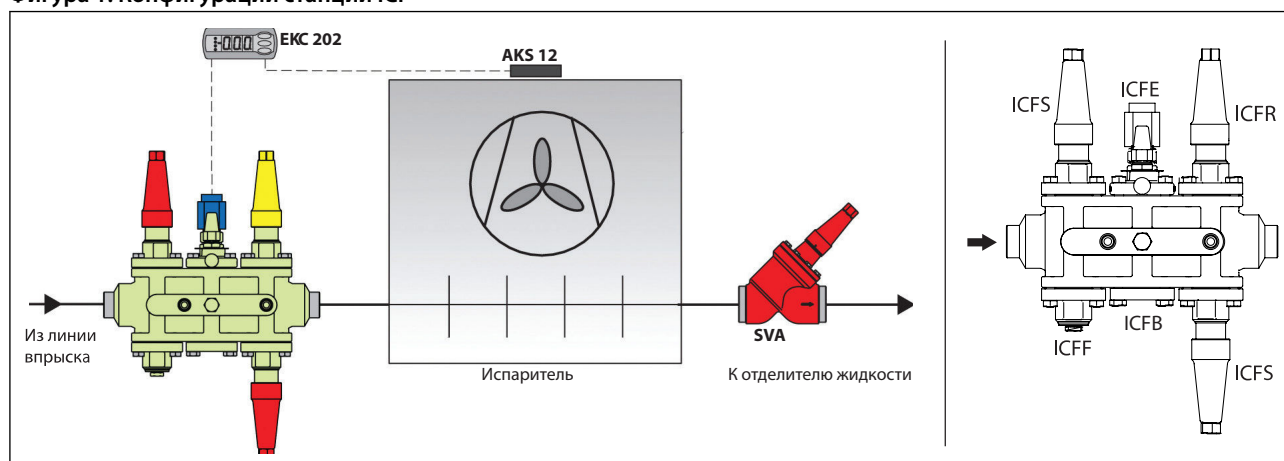
Фигура 1: Конфигурации станций ICF
