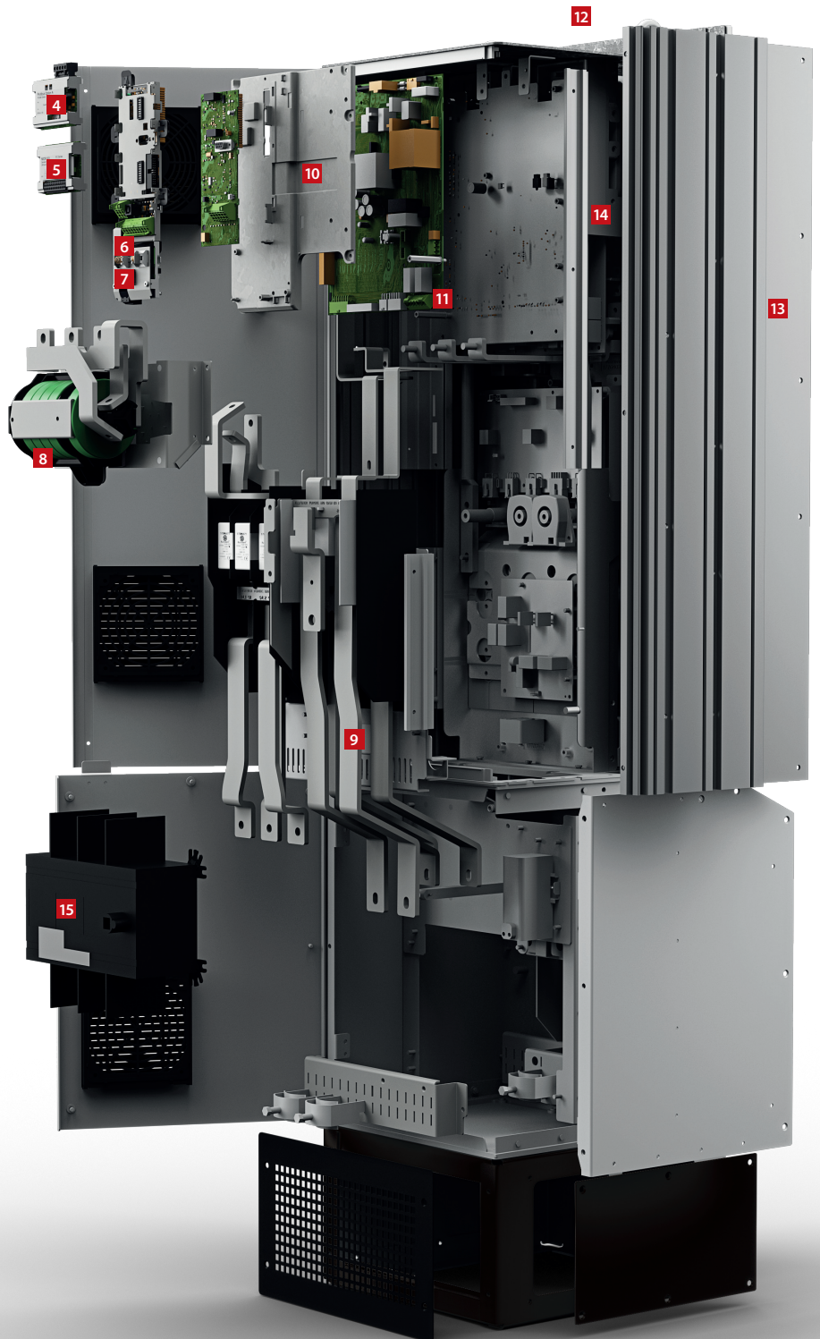
VLT® AutomationDrive FC 302, tamanho de gabinete T5
