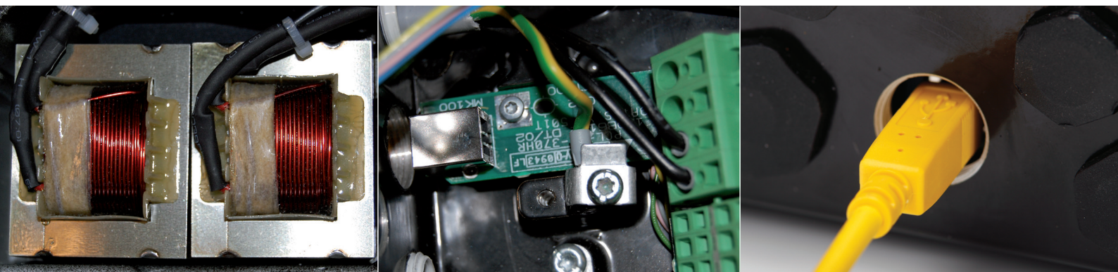
Beépített DC-tekercek a harmonikussterhítés korlátozásához
