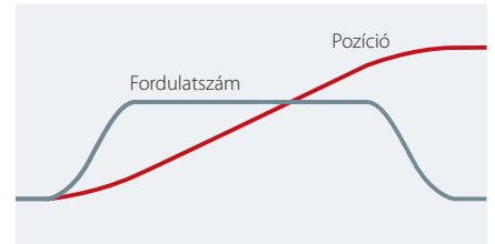
2. ábra. Mozcási profil S-rámpákkal
