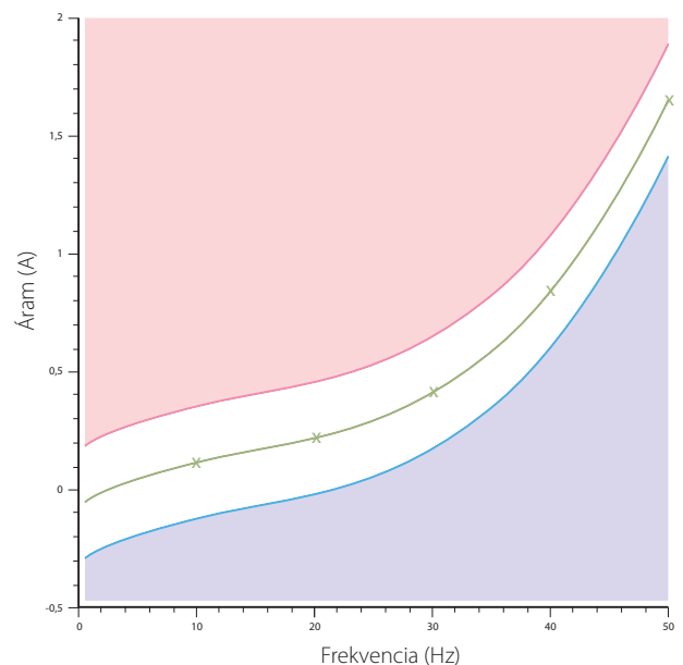
Alapérték – az energiafogyasztás terhelési burkológörbéjének felügyelete.
