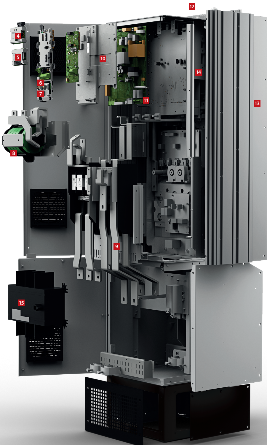
VLT® AutomationDrive FC 302, D5h házméret
