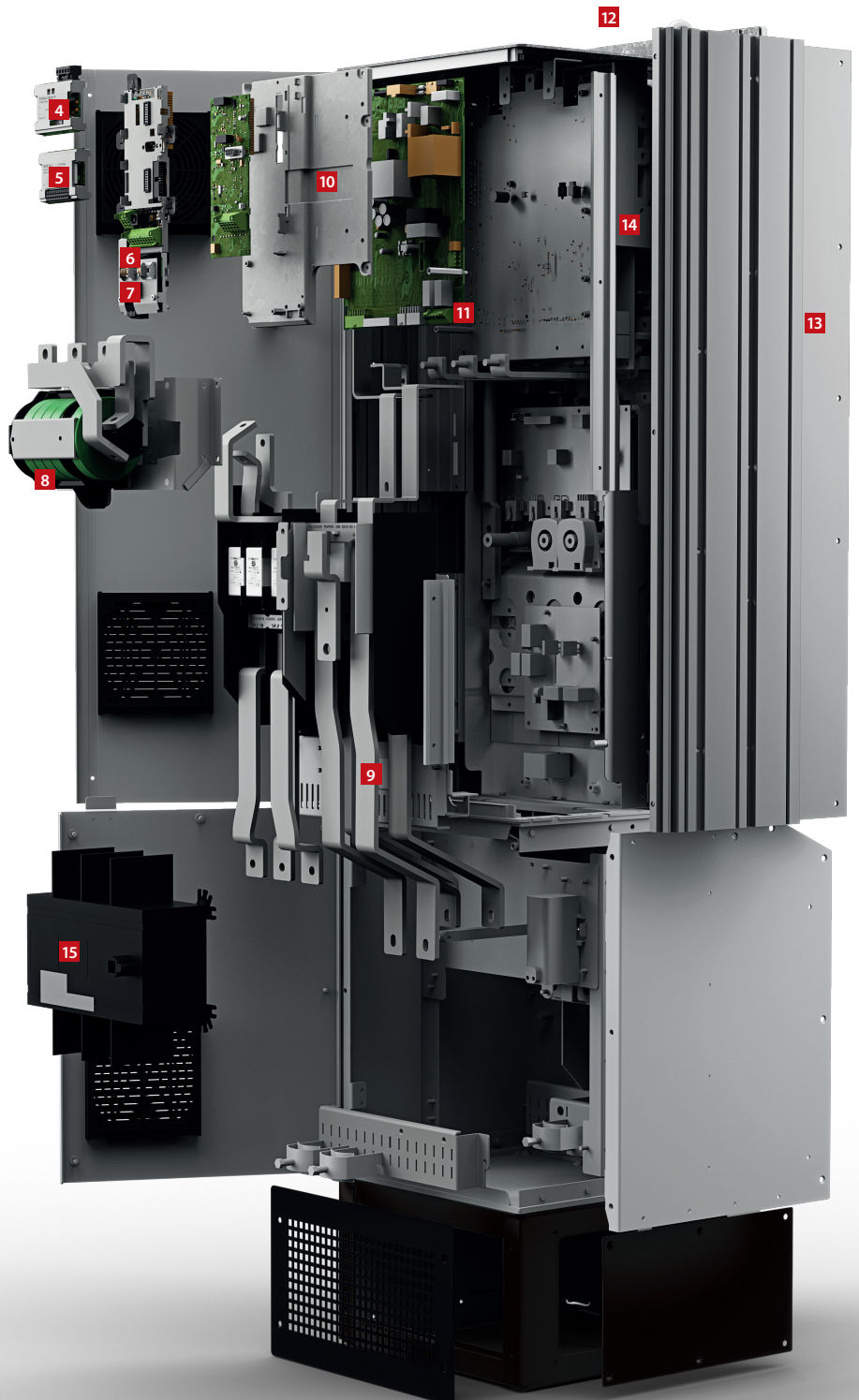
VLT® AutomationDrive FC 302, konstrukční velikost T5
