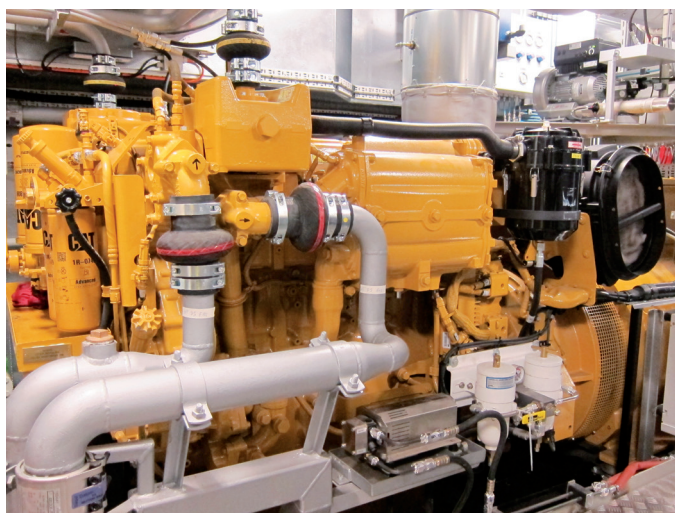
柴油电动发电机
