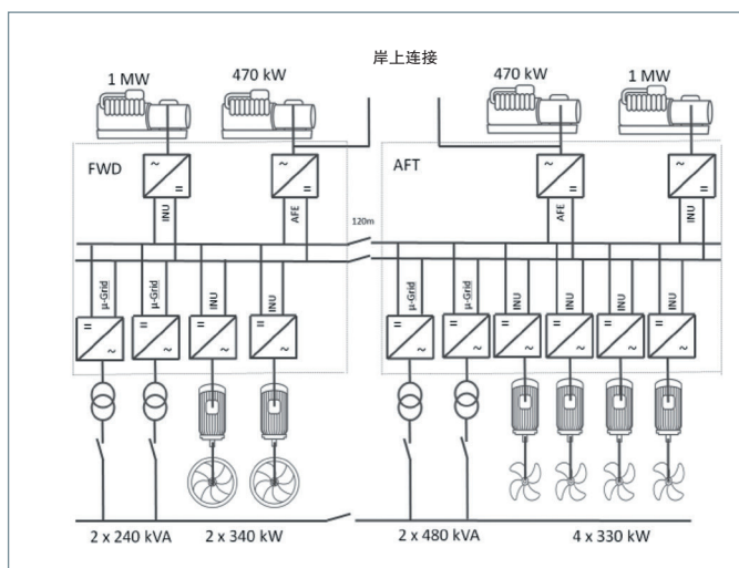
动力系统概览
