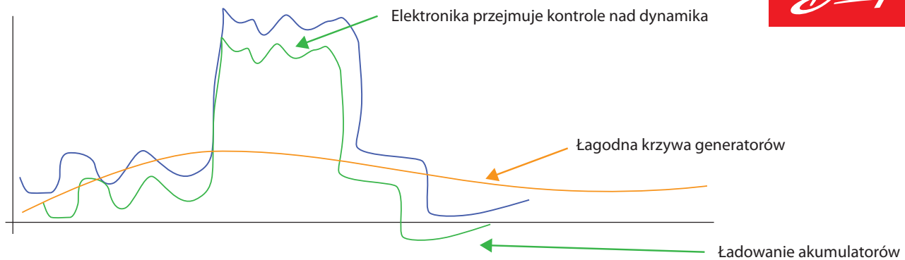
Ilustracja 4 Zarządzanie raptownymi zmianami za pośrednictwem elektronicznego systemu magazynowania.
