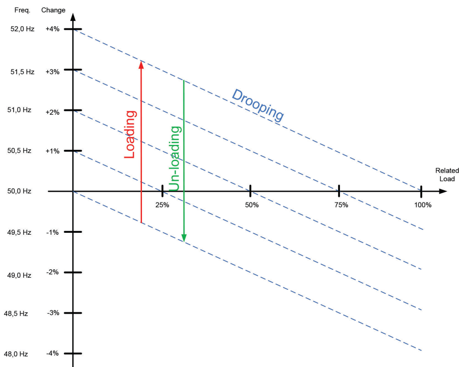
Ilustracja 5 Podział obciążenia.
