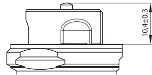
Stängningspunkt (mått) för DN 15–32
