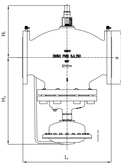
AB-QM DN 150
