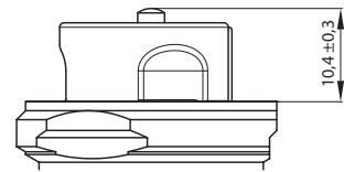
Sulgemispunkt (mõõtmine) ventiilile DN 15-32
