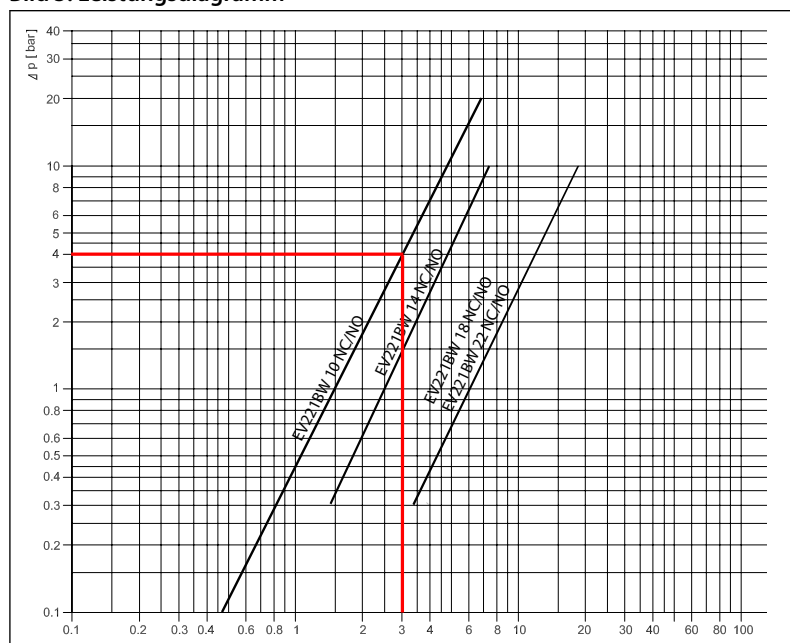
Bild 5: Leistungsdiagramm
