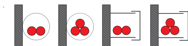
Método de instalación B1: conductores en un conducto o en cableado cerrado
