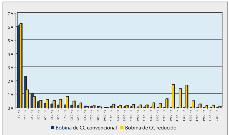
Los convertidores con bobinas de CC reducidas generan niveles armónicos más altos, especialmente en los intervalos de frecuencia más elevados.
