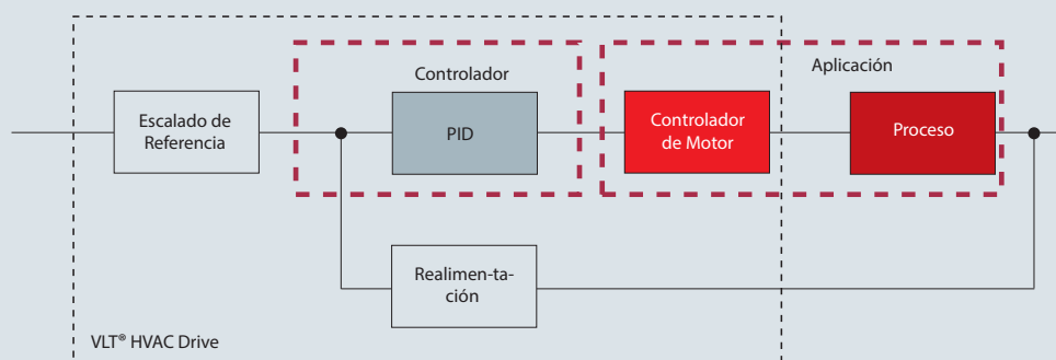
Diagrama de bloques del controlador de proceso PID
