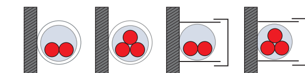
Método de instalación B2: cable multiconductor o cable apantallado multiconductor en un conducto o en cableado cerrado
