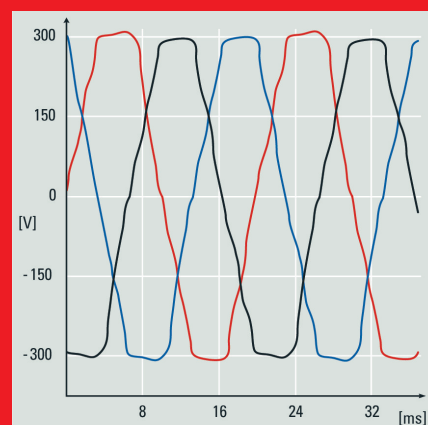
Oscylogram przedstawia wyraźne zniekształcenie napięcia sieci zasilającej spowodowane zakłóceniami pochodzącymi od obciążeń o charakterze nieliniowym
