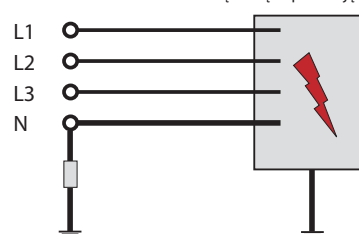
Układ zas. typu IT Układ izolowany od ziemi, bądź uziemiony poprzez dołączoną impedancję
