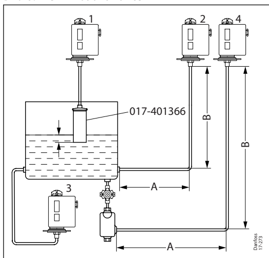
Bild 6: Vier Einbauvarianten
