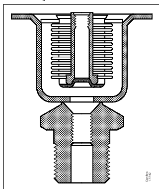
Bild 4: Querschnitt RT 32W
