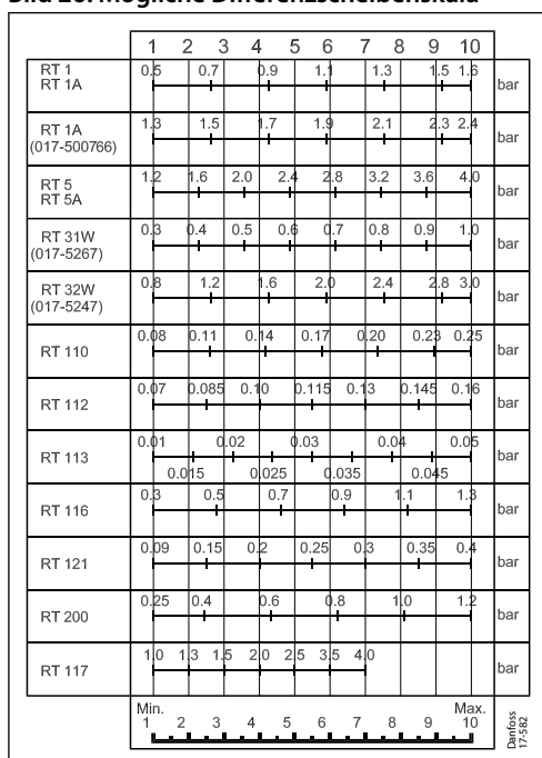
Bild 26: Mögliche Differenzscheibenskala
