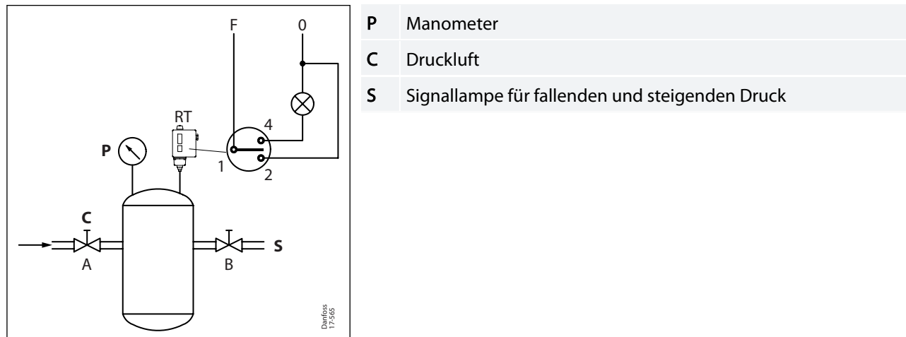
Bild 16: Testaufbau zum Einstellen des Druckschalters
