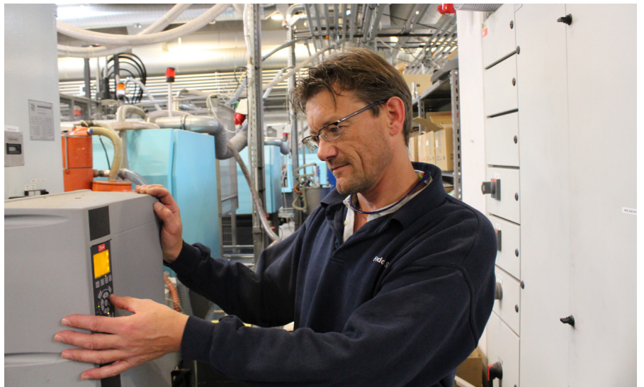
PTA-teamleder Freddy Søby ved en af de 55 kW frekvensomformere, der styrer sprøjtestøbemaskinerne.
