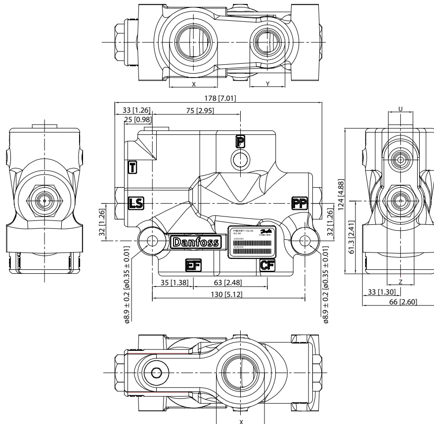
外形寸法とポート深さ
