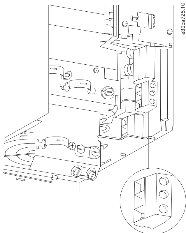
図 13: エンクロージャー・サイズ H10、IP20、600 V、11–15 kW (15–20 hp)
