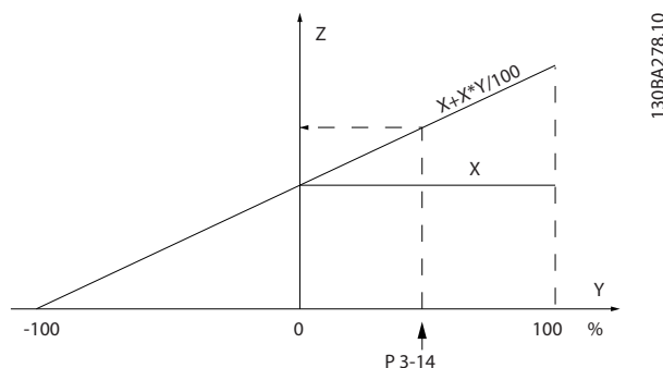
Ábra 3.20 Aktuális referencia
