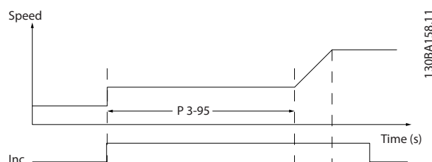
Ábra 3.25 Rámpa késleltetése, 1. eset
