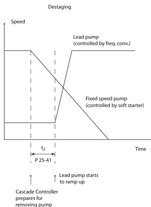
Ábra 3.91 Lekapcsolás
