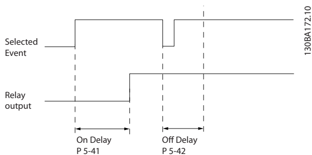
Ábra 3.30 Relékipacs. késlelt.
