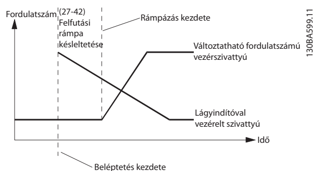
Ábra 3.108 Felfutási rámpa késleltetése
