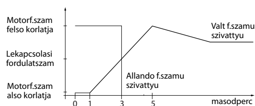
Ábra 3.93 Lekapcsolási küszöb
