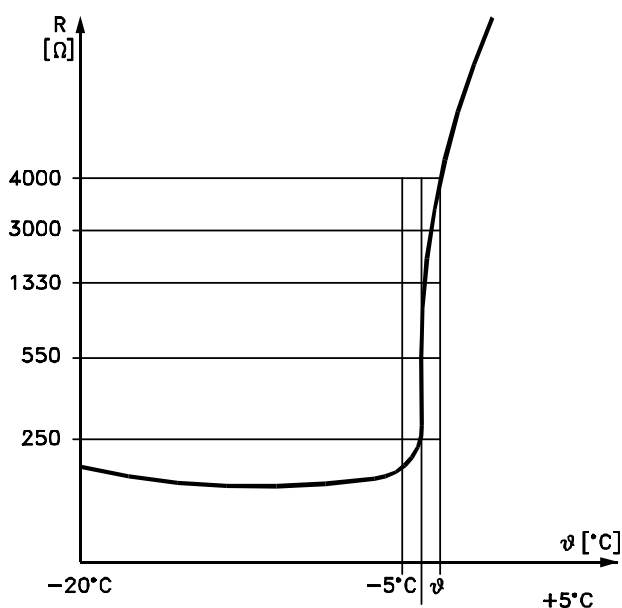
Ábra 3.12 PTC-profil
