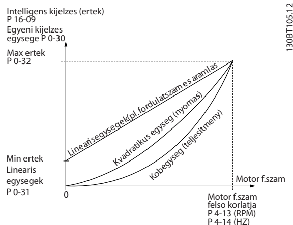
Ábra 3.3 Egyéni kijelzés
