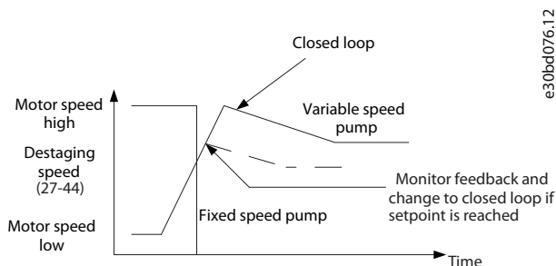
Ábra 3.110 Lekapcsolási küszöb
