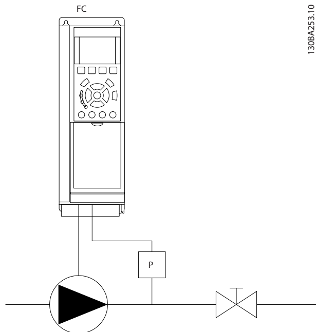
Ábra 3.64 Áramláshiány-észlelés rajza
