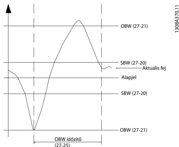
Ábra 3.88 Határsáv idő
