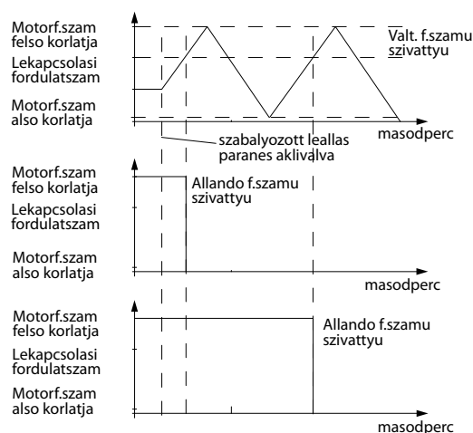
Ábra 3.94 Lekapcsolási fordulatszám
