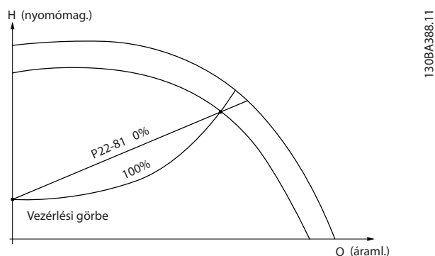
Ábra 3.71 Másodfokú-lineáris görbeközelítés
