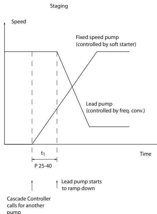
Ábra 3.90 Beléptetés
