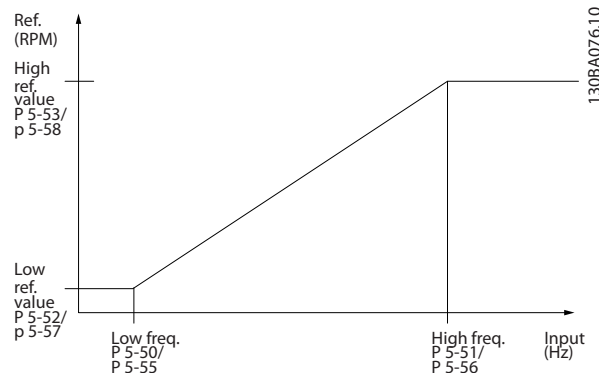
Ábra 3.31 Impulzusbemenet
