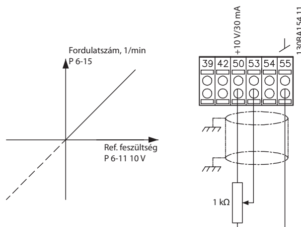
Ábra 1.9 Potenciométer-referencia
