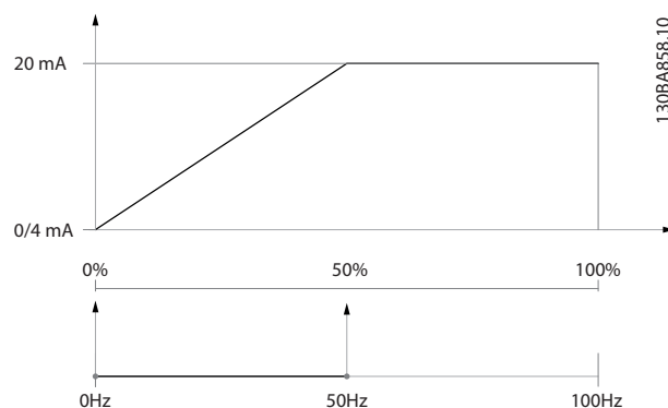
Ábra 3.37 1. példa
