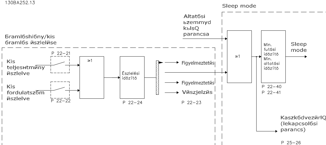
Ábra 3.63 Jelfolyamáb
