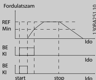
Ábra 3.28 A megkerülőszelep működési elve
