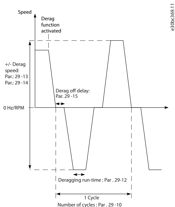
Ábra 3.114 Szivattyútisztítás funkció
