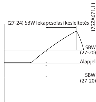
Ábra 3.106 Alapsáv lekapcsolási késleltetése
