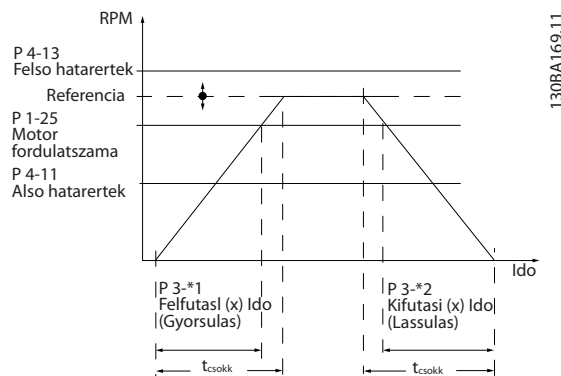
Ábra 3.21 1. rárpa
