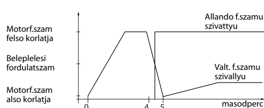
Ábra 3.92 Beléptetési küszöb
