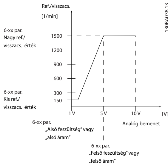
Ábra 3.34 Vezérlőjel-szakadási állapotok
