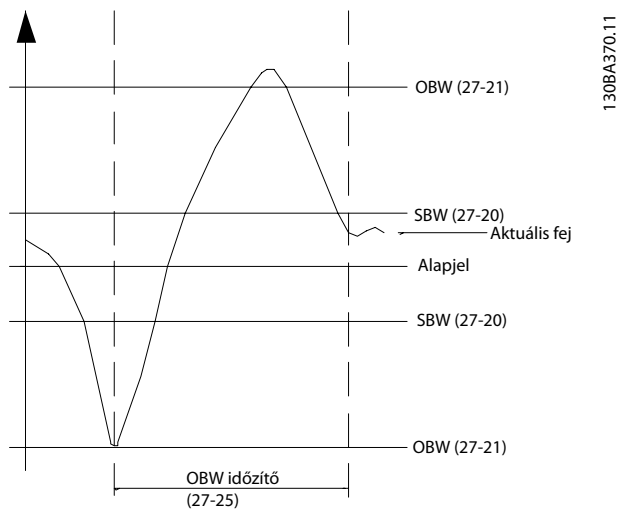
Ábra 3.101 Határsáv idő
