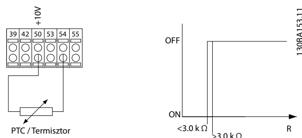
Ábra 3.14 PTC termisztor csatlakoztatása – analóg bemenet
