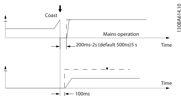
Ábra 3.96 Gyors konfiguráció
