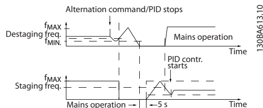
Ábra 3.95 Lassú konfiguráció
