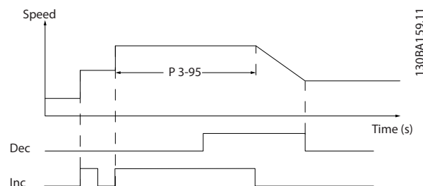
Ábra 3.26 Rámpa késleltetése, 2. eset
