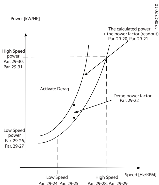
Ábra 3.115 Szivattyútisztítás teljesítményének beszabályozása
