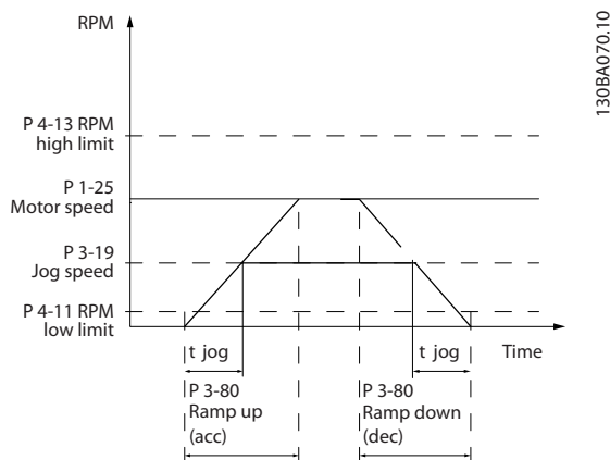
Ábra 3.22 Jográmpaidő
