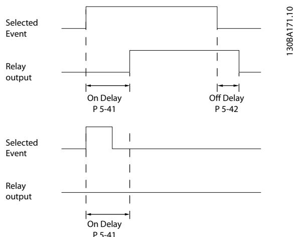
Ábra 3.29 Relébekapcsolás késleltetése
