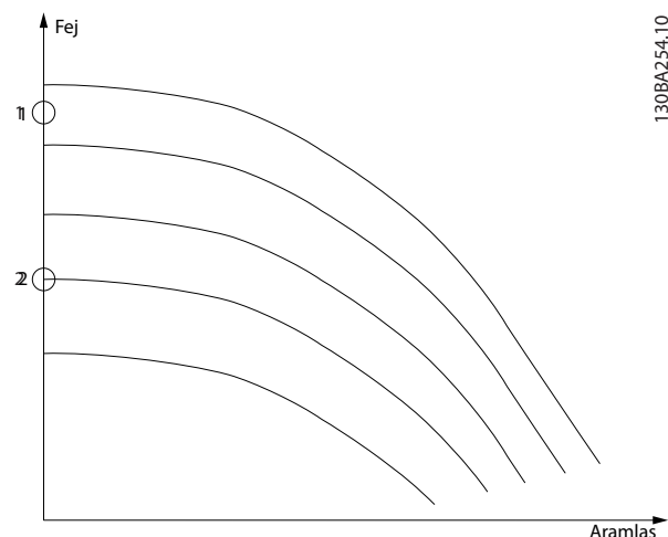
Ábra 3.65 Áramláshiány-észlelés diagramja
