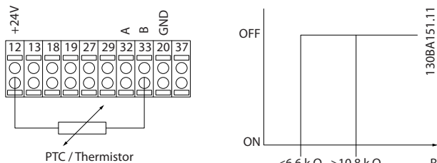
Ábra 3.16 Termisztor csatlakoztatása
