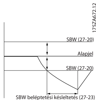
Ábra 3.102 Alapsáv beléptetési késleltetése
