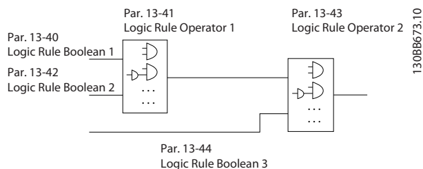
Ábra 3.44 Logikai szabályok
