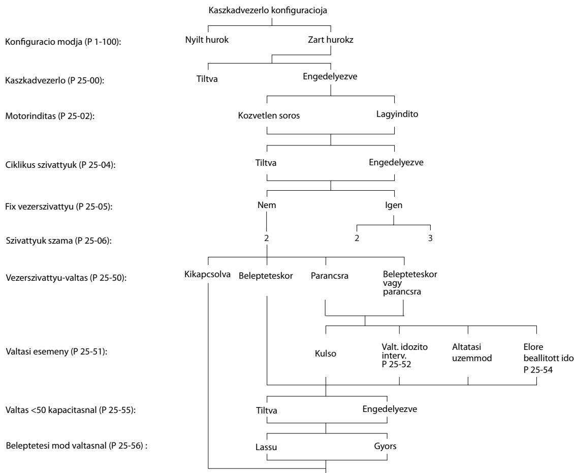
Ábra 3.79 Kaskádszabályozó beállítási példája
