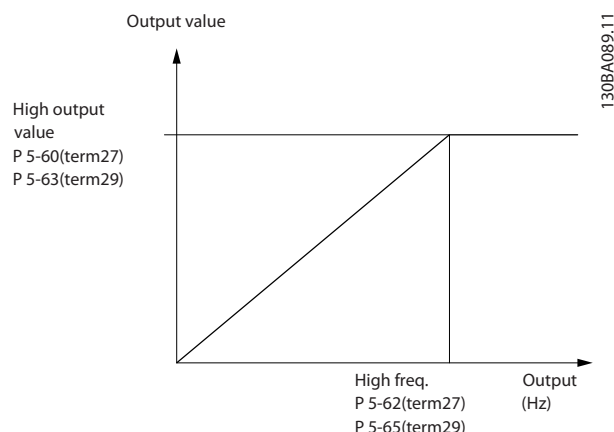
Ábra 3.32 Impulzuskimenet
