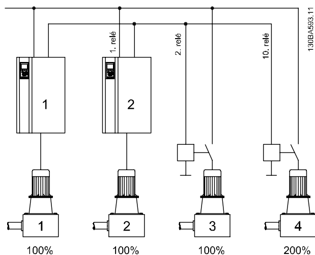
Ábra 3.98 Vegyes szivattyúkonfiguráció
