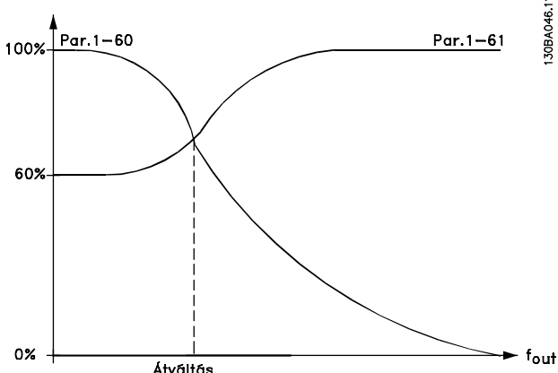
Ábra 3.10 TerheléskompENZáció kis fordulatszám
