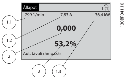
Ábra 2.11 I. állapotképernyő
