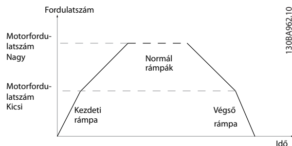
Ábra 3.23 Kezdeti és végso rámpaidő
