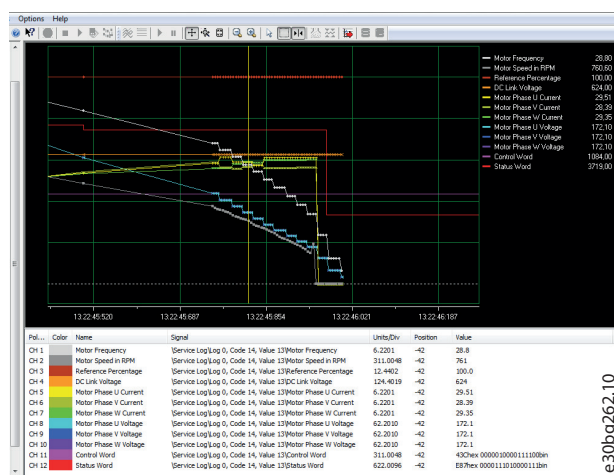
Ábra 3.58 Részletes szerviznaplónézet, 250 ms
