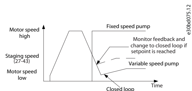
Ábra 3.109 Beléptetési küszöb
