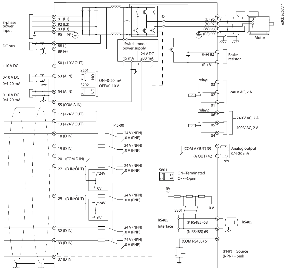
Ábra 1.2 Alapvető bekötési rajz
