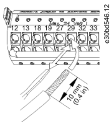
Ilustración 36: Conexión de un cable de control flexible a la caja de terminales
