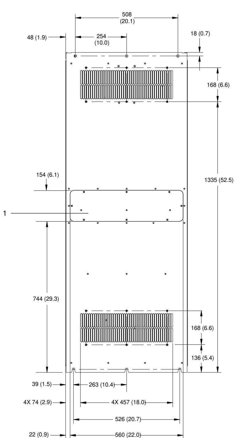
Ilustración 66: Vista posterior del alojamiento E4h
