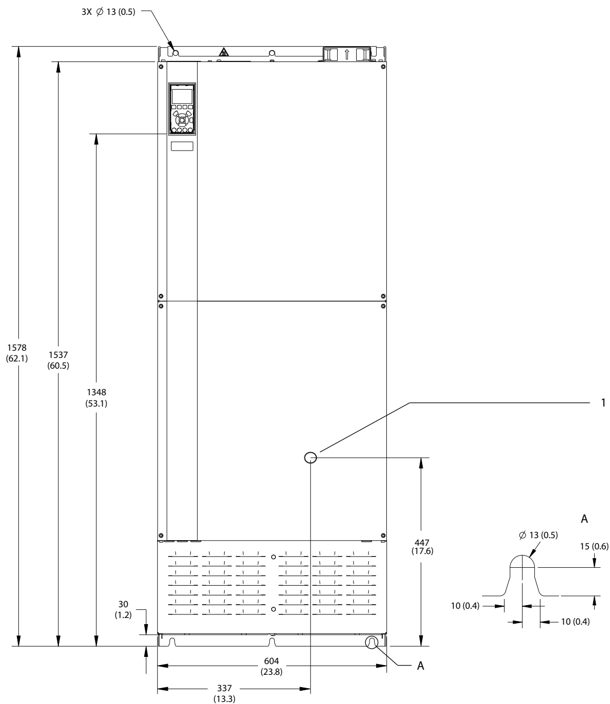
Ilustración 64: Vista frontal del alojamiento E4h
