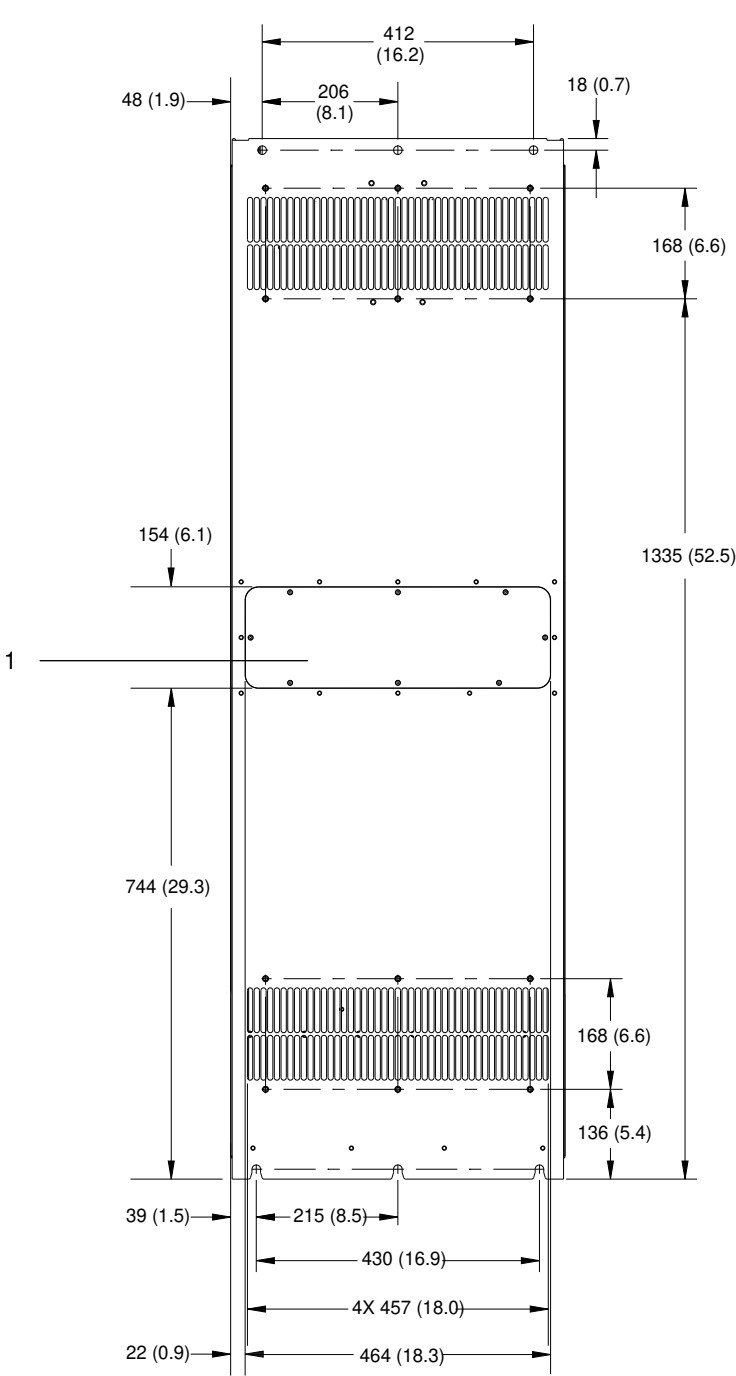
Ilustración 62: Vista posterior del alojamiento E3h
