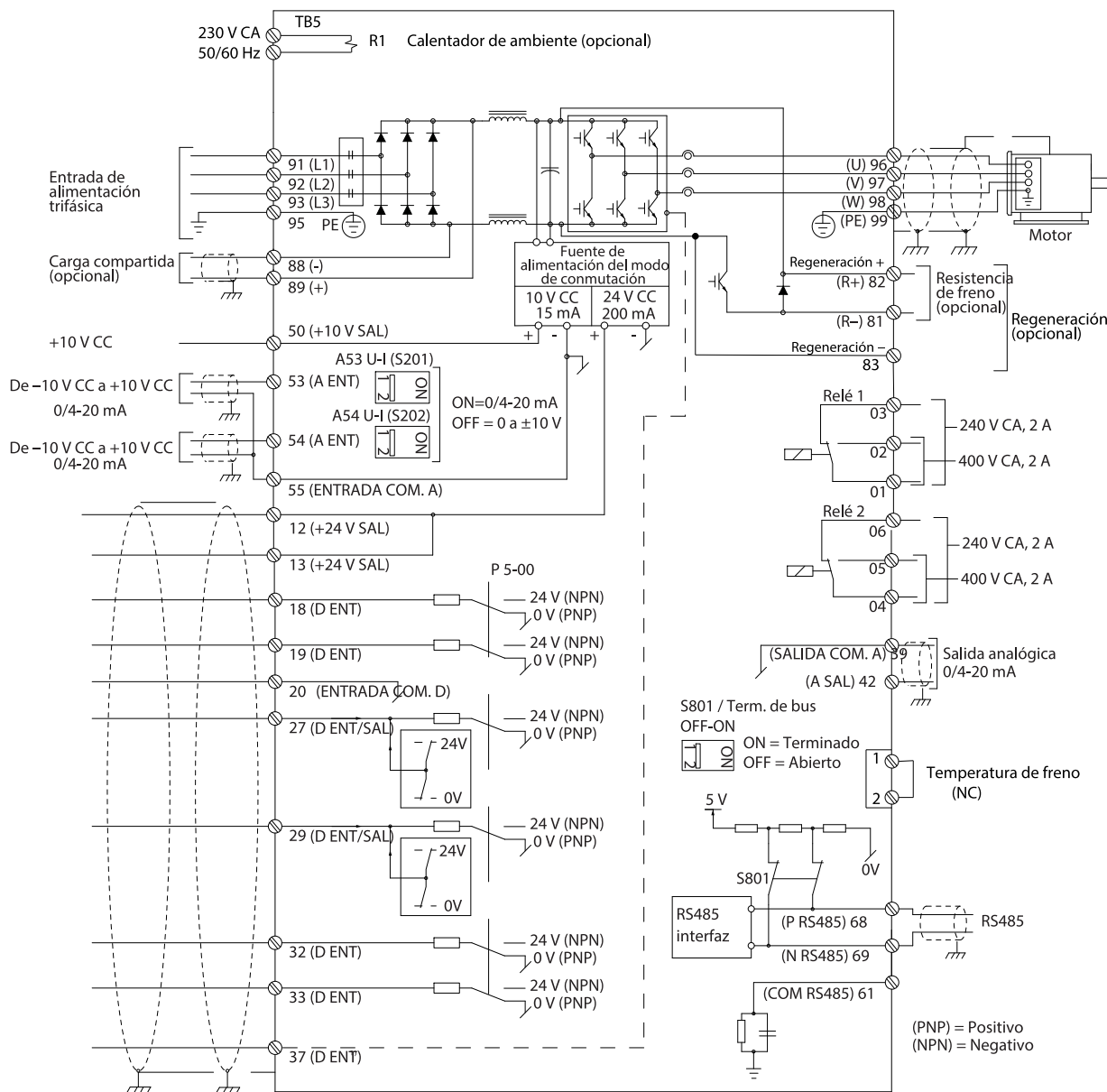
Ilustración 17: Esquema básico del cableado
