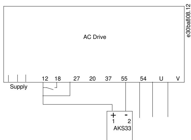
Ilustración 46: Modo de conexión de las unidades FC 103 y AKS33 para aplicaciones de lazo cerrado
