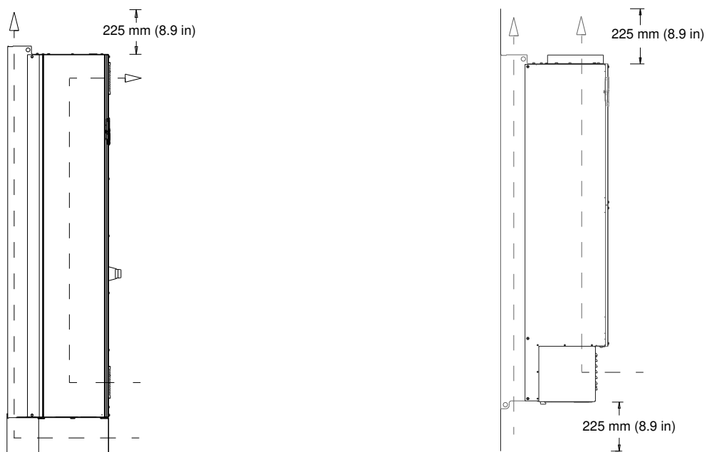
Ilustración 68: Flujo de aire para E1h/E2h (izquierda) y E3h/E4h (derecha)
