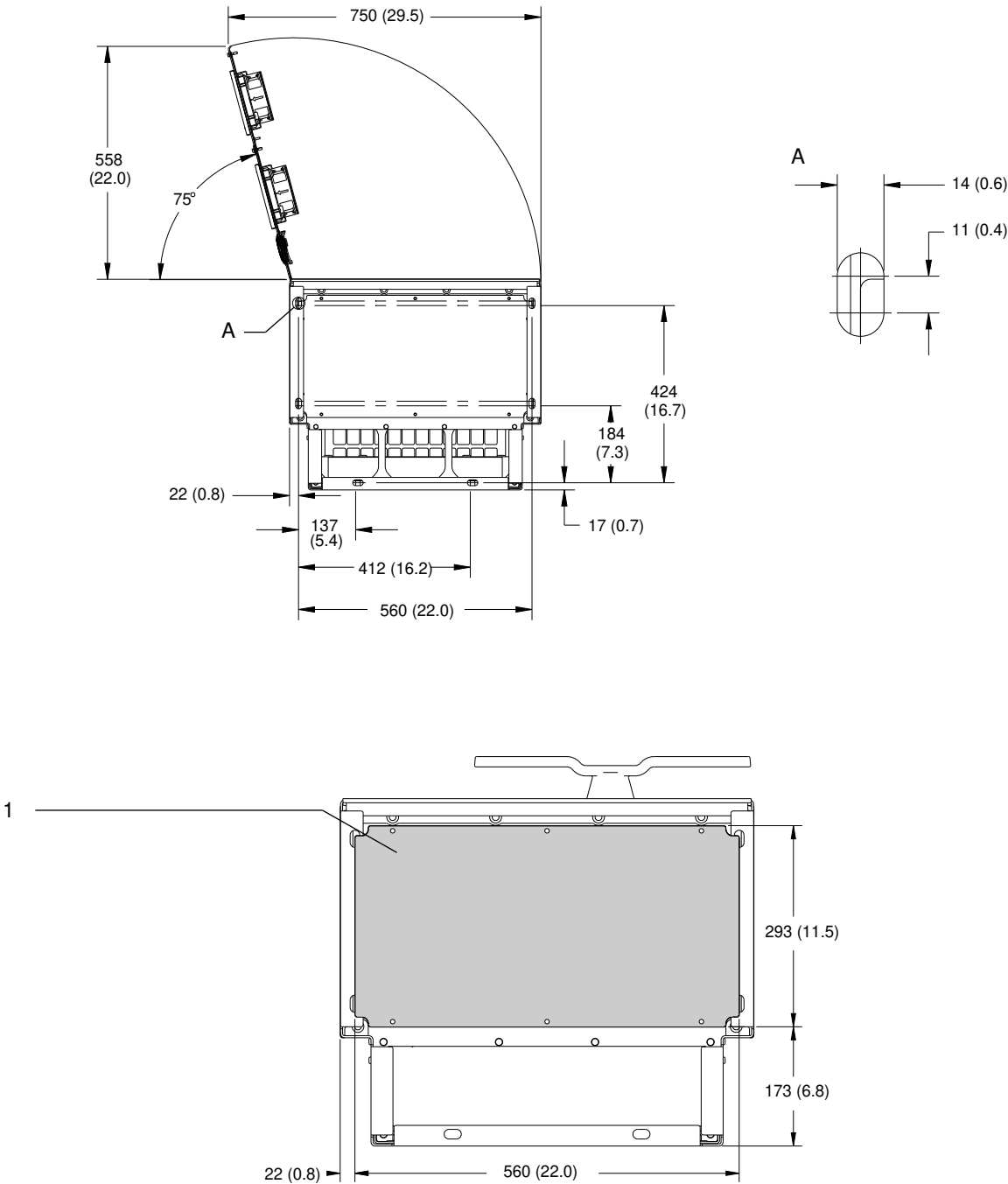
Ilustración 55: Dimensiones de la placa de entrada de cables y del espacio libre para la puerta del alojamiento E1h
