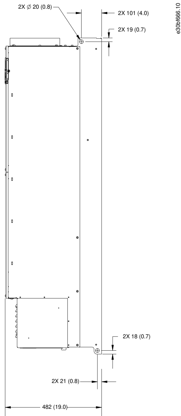
Ilustración 65: Vista lateral del alojamiento E4h
