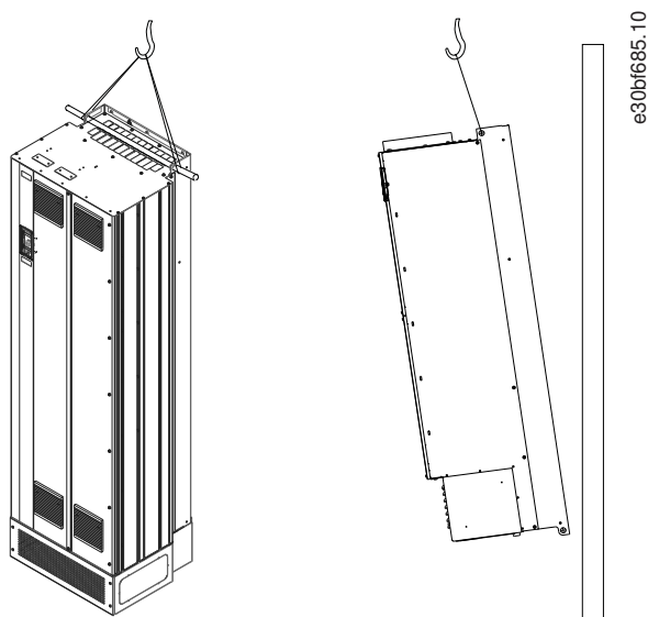
Ilustración 8: Método recomendado de elevación
