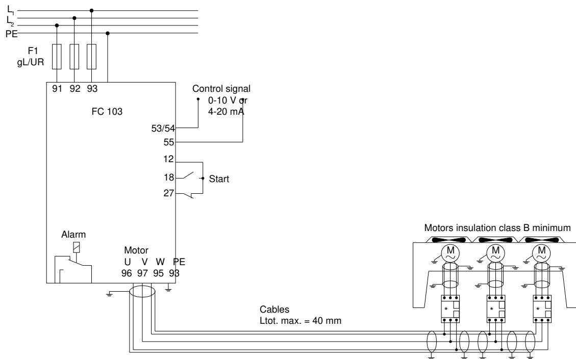
Ilustración 43: Control de velocidad con referencia analógica (lazo abierto). Bomba o ventilador único, o varios ventiladores o bombas en paralelo.
