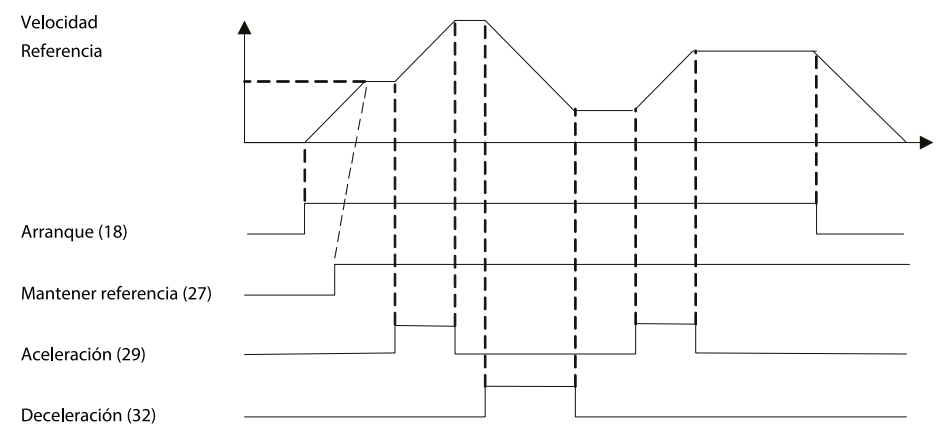
Ilustración 39: Aceleración/deceleración
