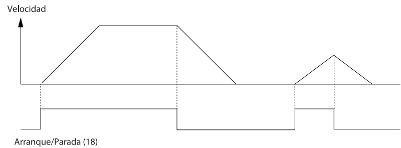
Ilustración 40: Orden de arranque/parada con Safe Torque Off
