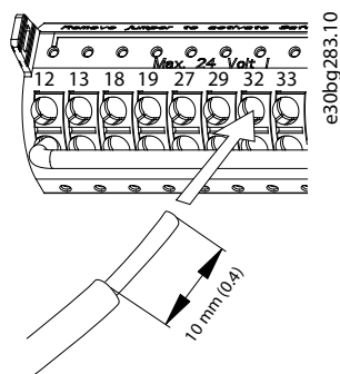
Ilustración 35: Conexión de un cable de control sólido a la caja de terminales
