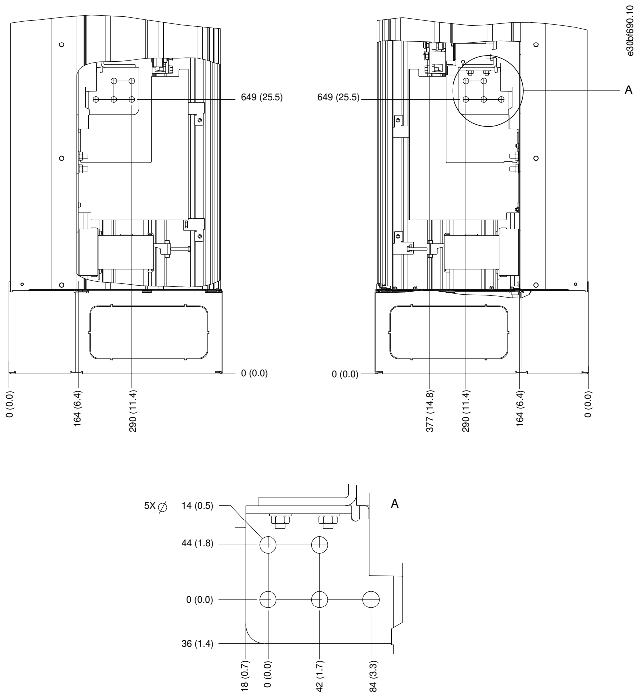
Ilustración 24: Dimensiones de los terminales del alojamiento E2h (vistas laterales)
