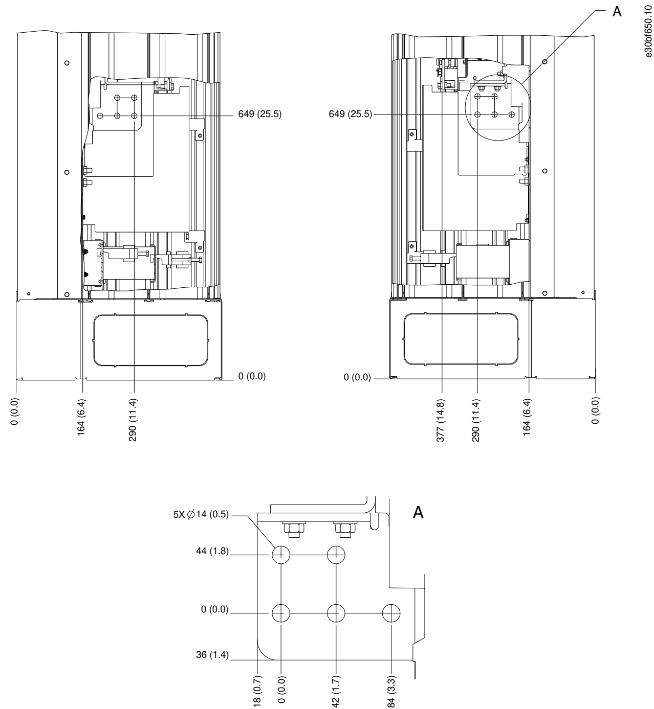
Ilustración 22: Dimensiones de los terminales del alojamiento E1h (vistas laterales)
