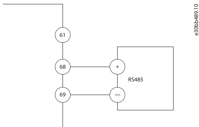
Ilustración 37: Diagrama de cableado de comunicación serie
