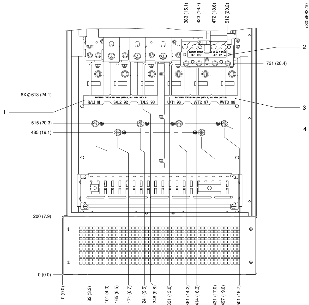
Ilustración 21: Dimensiones de los terminales del alojamiento E1h (vista frontal)
