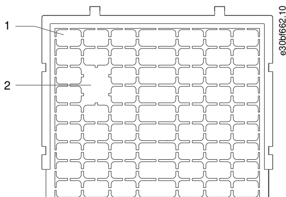
Ilustración 13: Placa de entrada de cables de plástico
