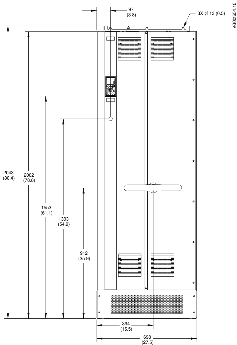
Ilustración 56: Vista frontal del alojamiento E2h
