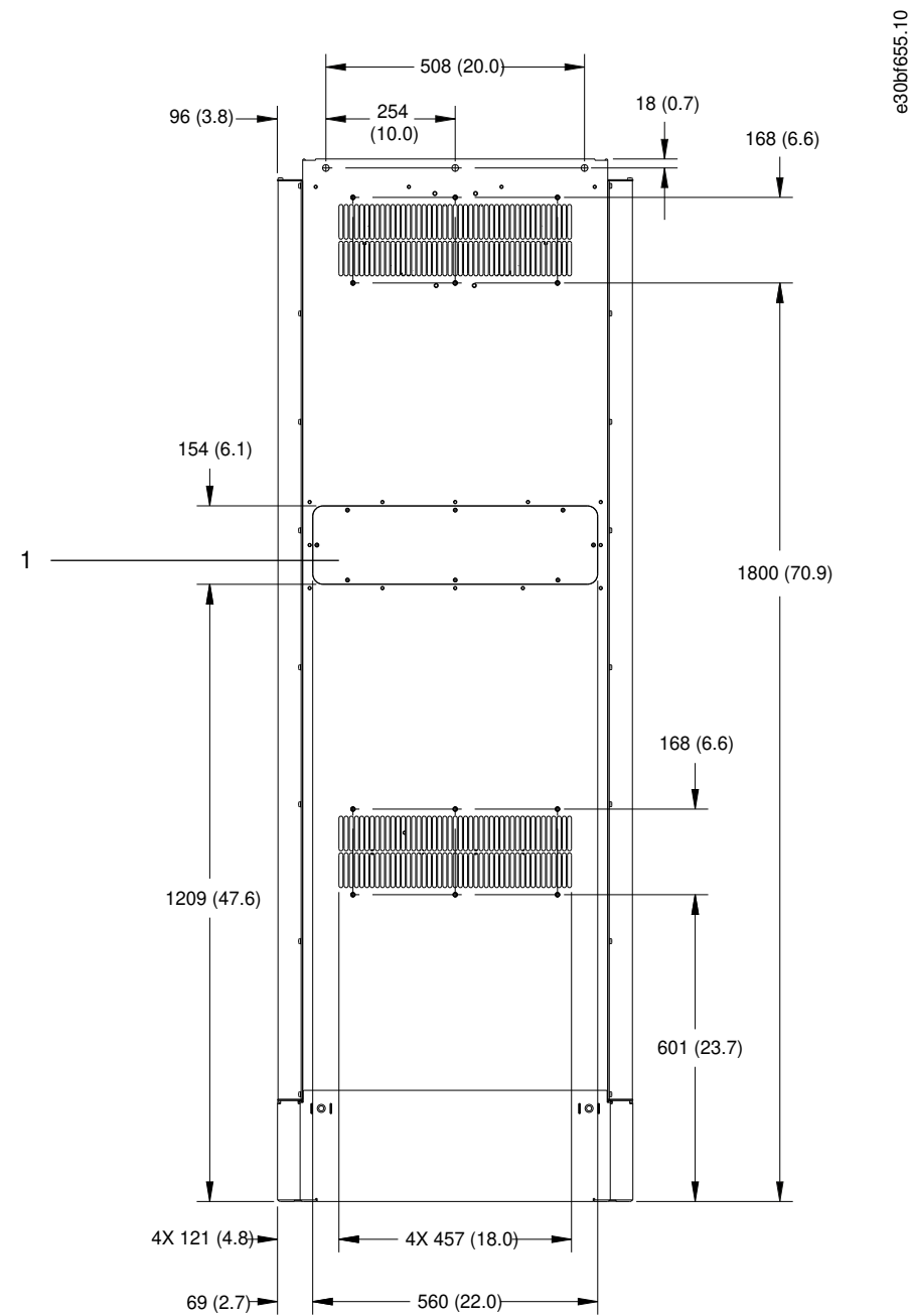
Ilustración 58: Vista posterior del alojamiento E2h
