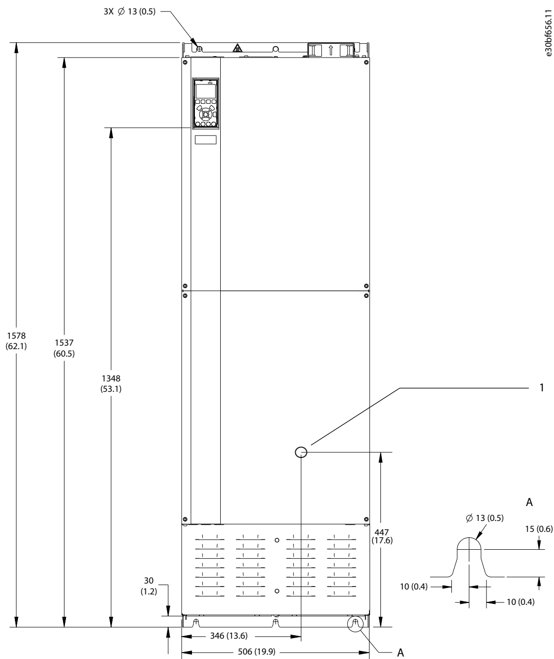
Ilustración 60: Vista frontal del alojamiento E3h
