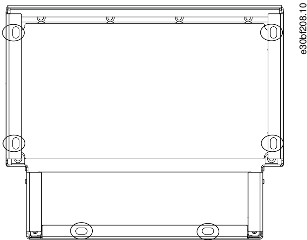
Ilustración 9: Puntos de montaje en el suelo del pedestal (indicados con un círculo).
