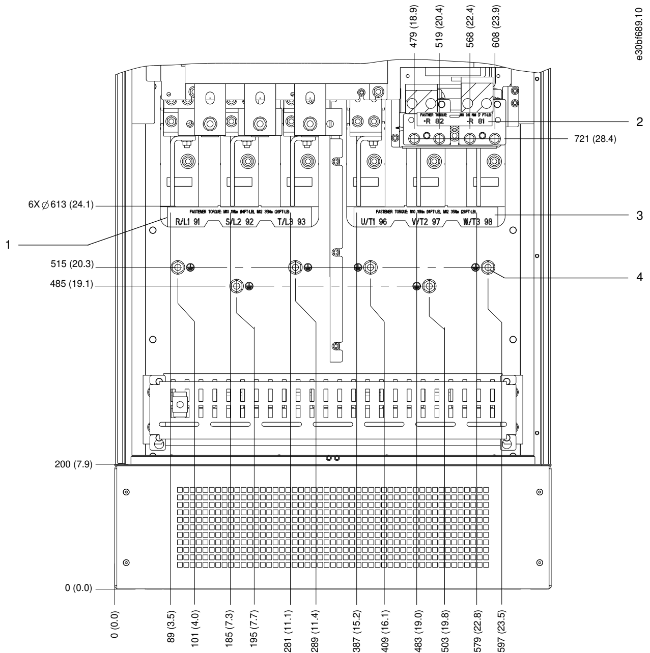
Ilustración 23: Dimensiones de los terminales del alojamiento E2h (vista frontal)
