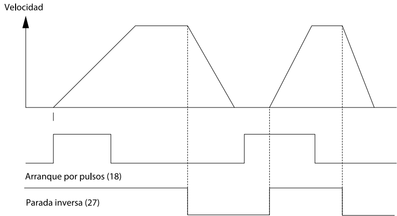
Ilustración 41: Arranque por pulsos / parada inversa
