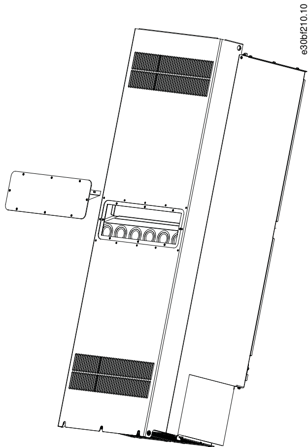
Ilustración 47: Panel de acceso al disipador extraído desde la parte trasera del convertidor
