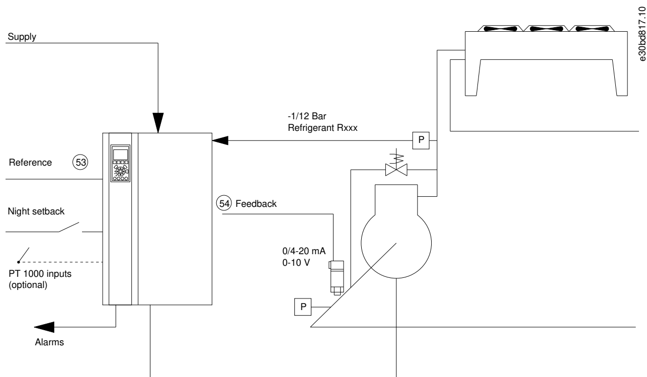
Ilustración 42: Configuración estándar del «Compresor con control interno»
