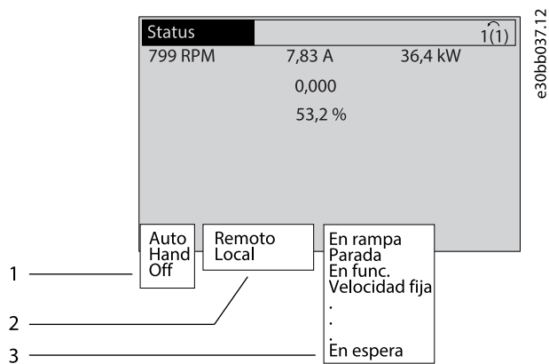
Ilustración 48: Pantalla de estado
