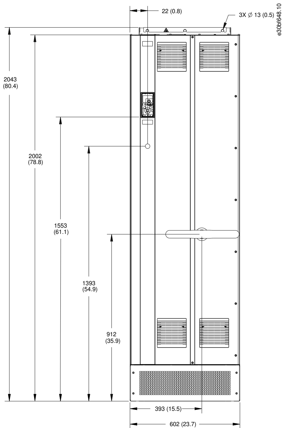
Ilustración 52: Vista frontal del alojamiento E1h
