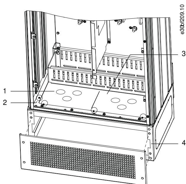
Ilustración 12: Instalación de la placa de entrada de cables
