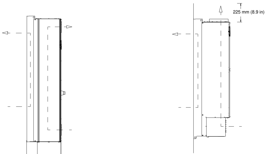
Ilustración 69: Flujo de aire con kits de refrigeración de pared posterior en E1h/E2h (izquierda) y E3h/E4h (derecha)
