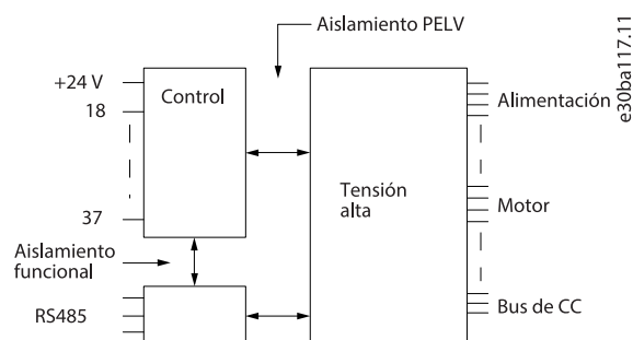
Ilustración 51: Aislamiento PELV
