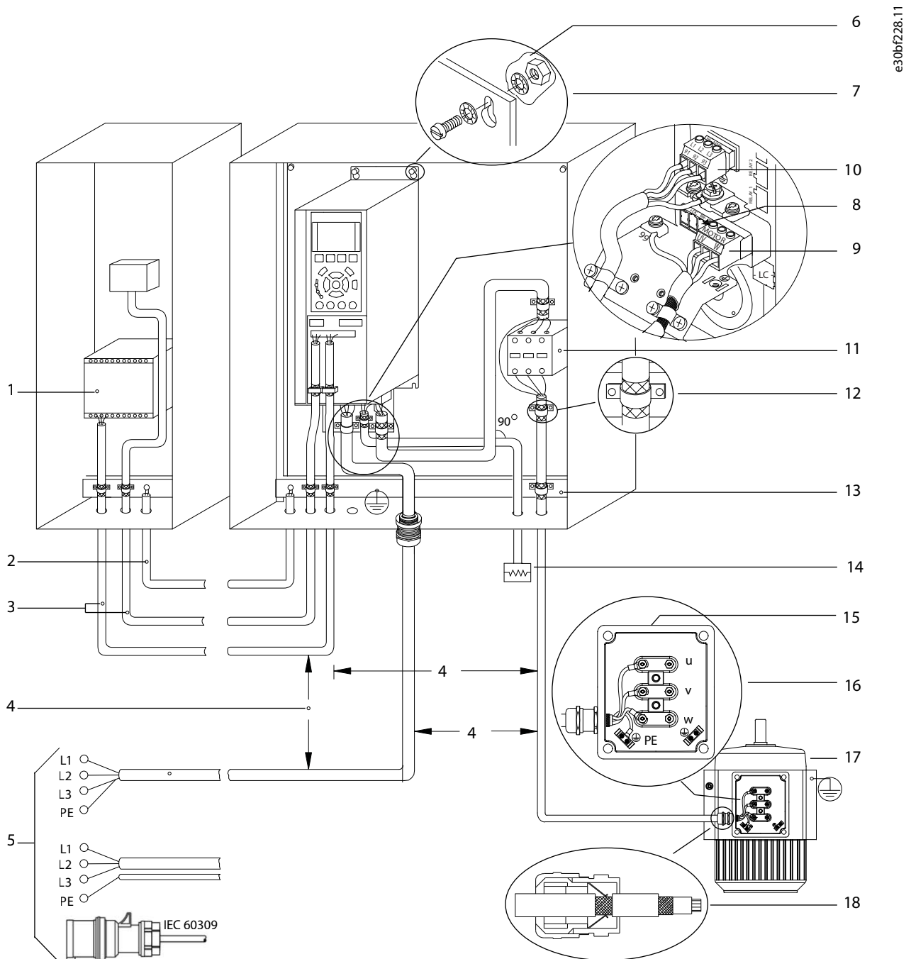
Ilustración 16: Ejemplo de instalación correcta en cuanto a EMC
