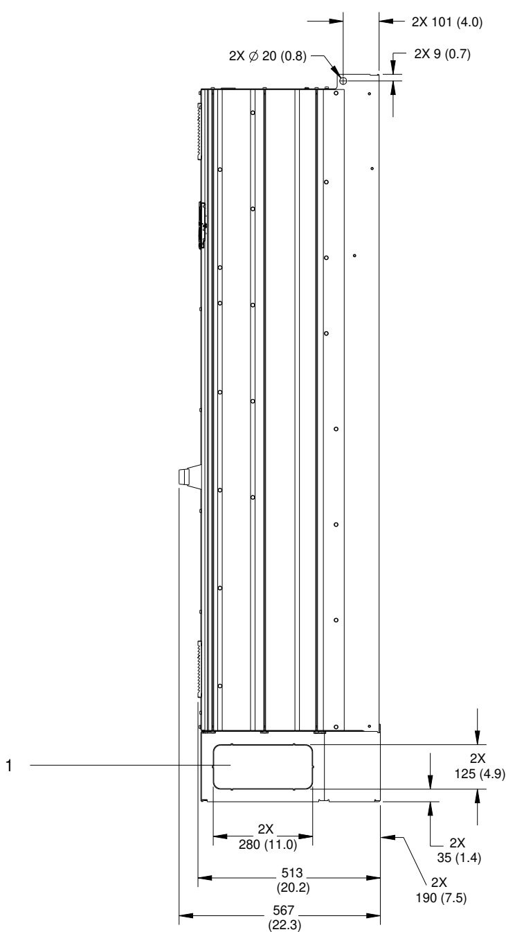
Ilustración 57: Vista lateral del alojamiento E2h
