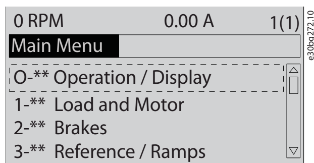
Ábra 6.2 A főmenü
