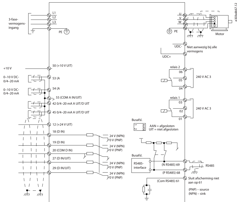
Afbeelding 25: Eenvoudig bedradingschema
