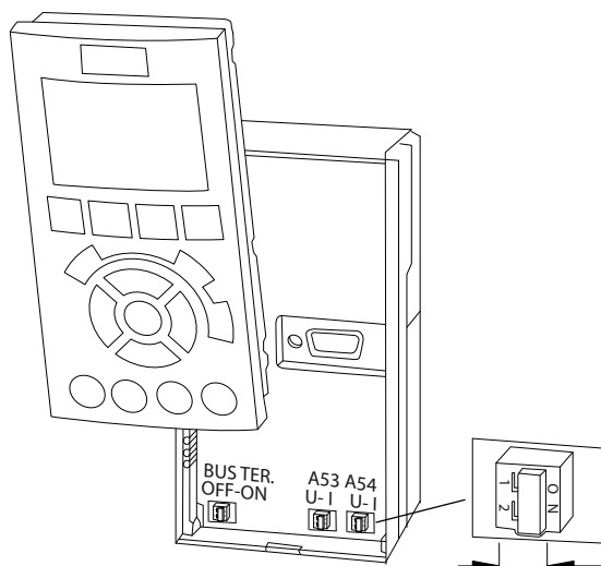
Ilustracja 5.23 Położenie przełączników zacisków 53 i 54
