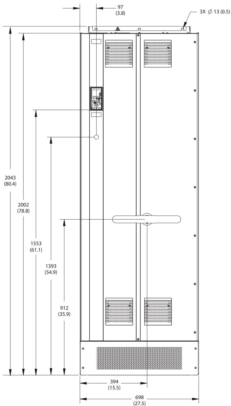
Ilustracja 9.6 E2h, widok z przodu
