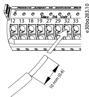
Ilustracja 5.20 Podłączanie jednodrutowych przewodów sterowania
