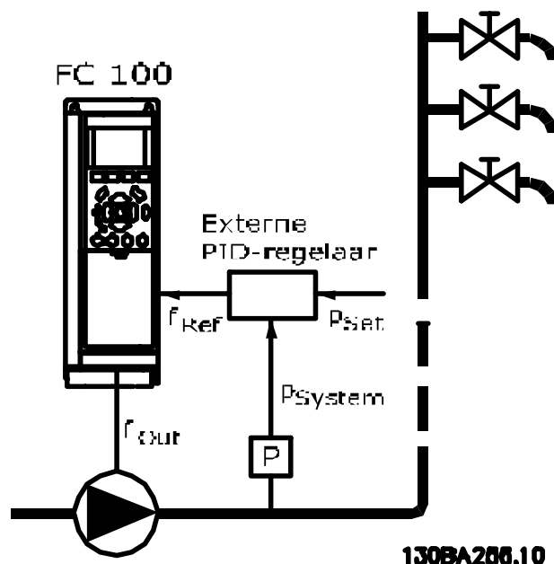
Afbeelding 3.68 Systeem met drukterugkoppeling
