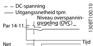
Afbeelding 3.52 Kinetische backup, korte netstoring
