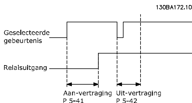
Afbeelding 3.30 Uit-vertr., relais
