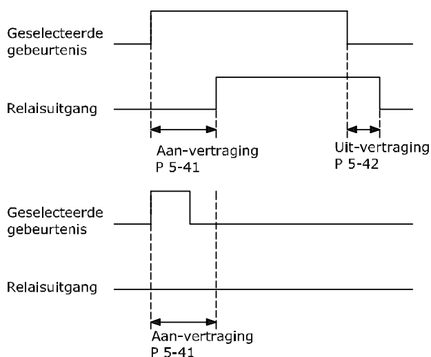
Afbeelding 3.29 Aan-vertr., relais
