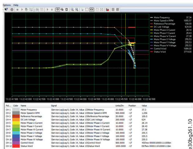
Afbeelding 3.57 Servicelogweergave, 5 s
