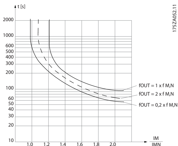
Afbeelding 3.15 ETR-profiel
