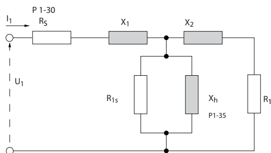
Afbeelding 3.4 Motorequivalentiediagram voor een asynchrone motor
