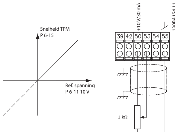
Afbeelding 1.9 Potentiometerreferentie
