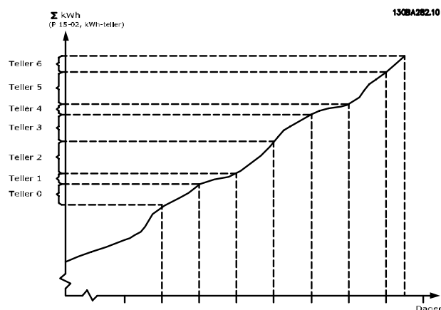
Afbeelding 3.75 Grafiek energielog
