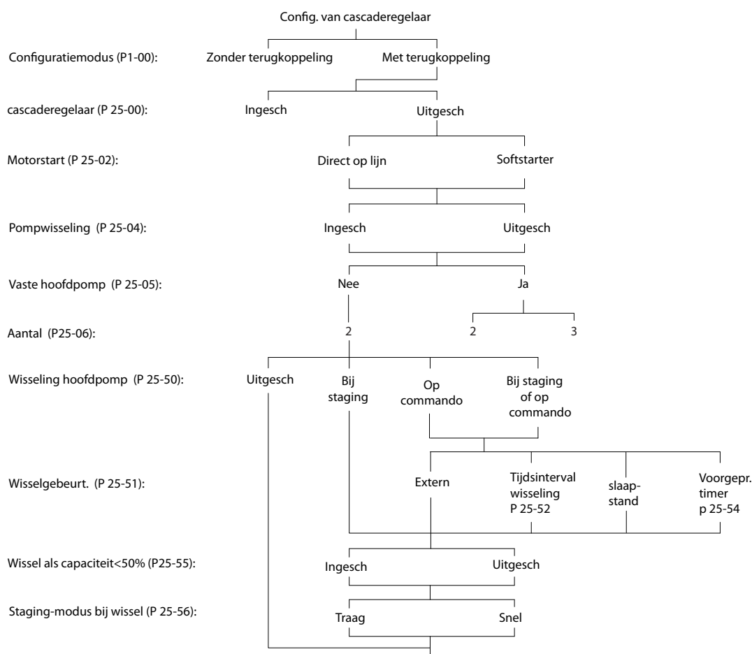
Afbeelding 3.79 Voorbeeldsetup cascaderegelaar
