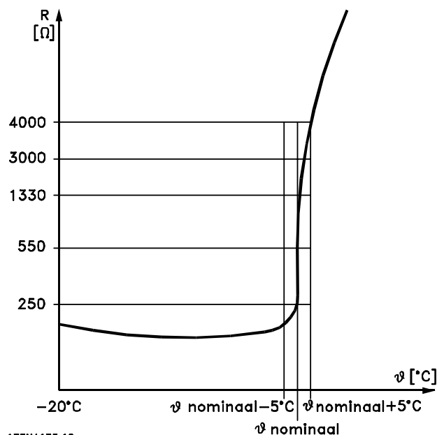
Afbeelding 3.12 PTC-profiel
