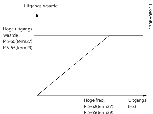
Afbeelding 3.32 Pulsuitgang
