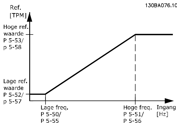
Afbeelding 3.31 Pulsingang
