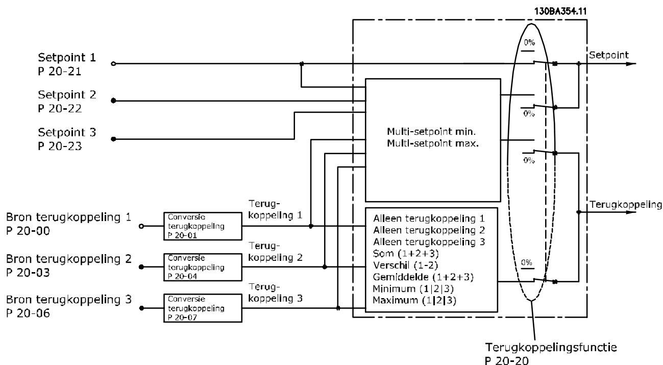
Afbeelding 3.60 Ingangssignalen in PID-terugkoppelingsregelaar.
