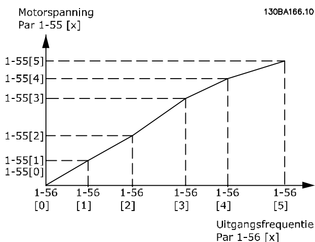
Afbeelding 3.9 U/f-karakteristiek
