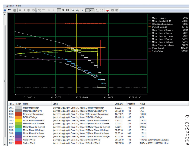
Afbeelding 3.58 Servicelogweergave, 250 ms
