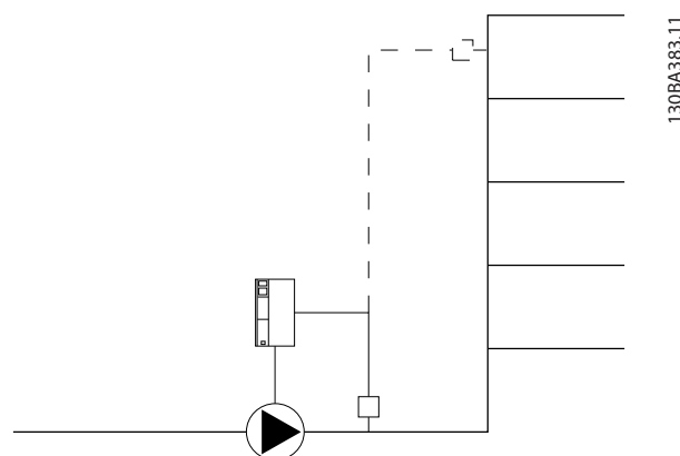
Afbeelding 3.70 Setup flowcompensatie
