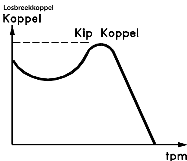
Afbeelding 1.1 Losbreekkoppel
