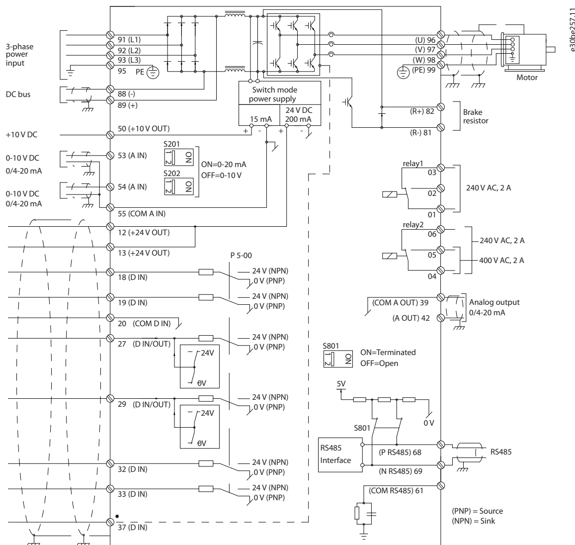
Afbeelding 1.2 Eenvoudig bedradingsschema
