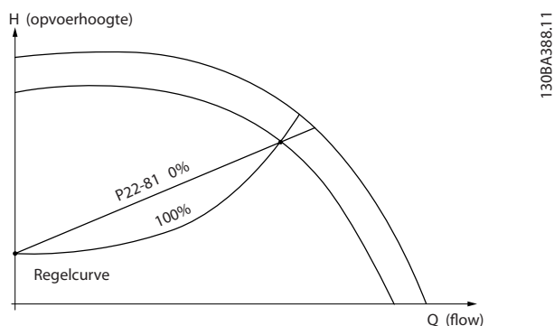
Afbeelding 3.71 Kwadr-lineaire curvebenadering
