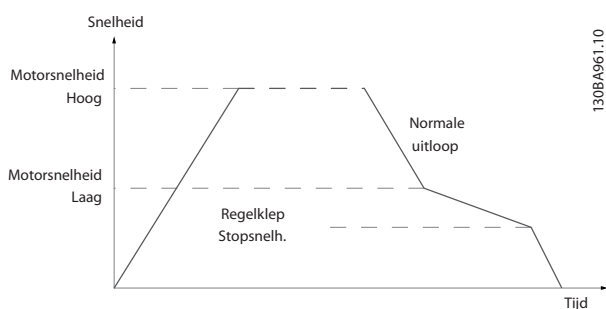
Afbeelding 3.24 Uitloop terugslagklep
