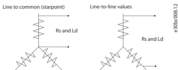
Afbeelding 3.6 Statorwikkelingconfiguraties
