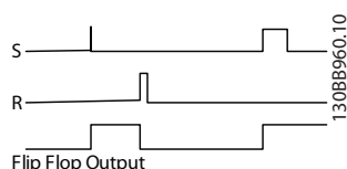
Afbeelding 3.43 Flip-flopuitgangen
