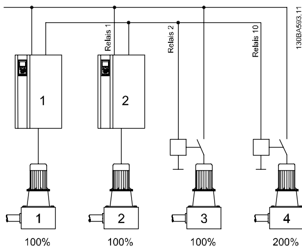
Afbeelding 3.96 Gemengde-pompconfiguratie
