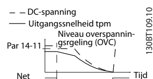
Afbeelding 3.53 Kinetische backup, langere netstoring
