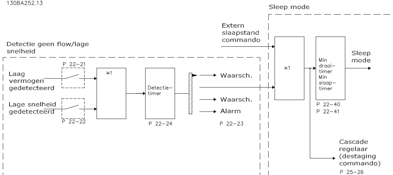
Afbeelding 3.63 Signaal-flowschema
