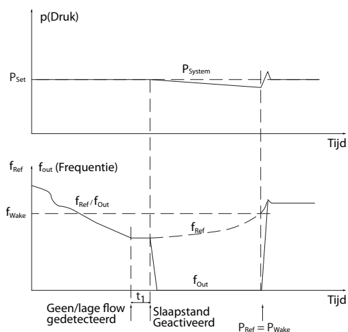
Afbeelding 3.69 Booststelsel zonder drukterugkoppeling
