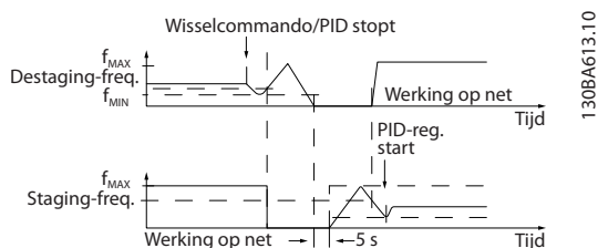
Afbeelding 3.93 Trage configuratie
