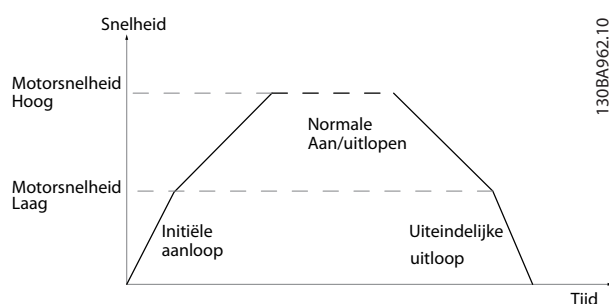
Afbeelding 3.23 Initiële en uiteindelijke ramp-tijd
