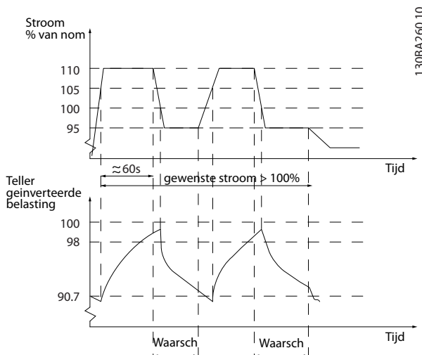
Afbeelding 3.55 Uitgangsstroom bij overbelasting
