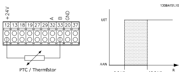
Afbeelding 3.16 Aansluiting thermistor
