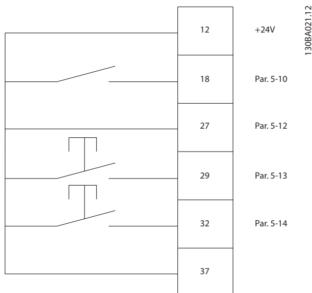
Afbeelding 1.8 Snelheid omhoog/omlaag
