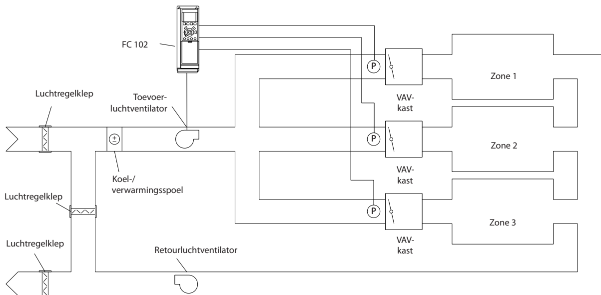
Afbeelding 3.61 Toepassingsschema multizone
