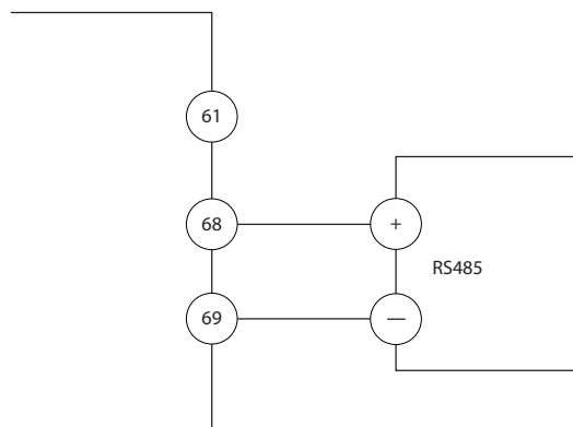
Ilustrația 5.22 Diagrama de cablare pentru comunicația serială
