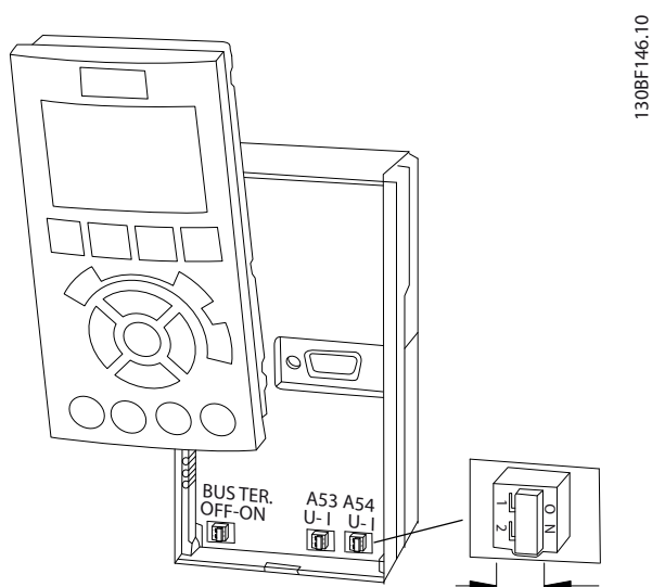
Ilustrația 5.23 Locația comutatoarelor bornelor 53 și 54
