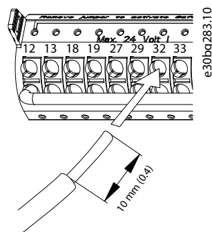
Ilustrația 5.20 Conectarea conductorilor de control solizi
