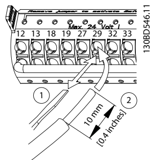
Ilustrația 5.21 Conectarea conductorilor de control flexibili
