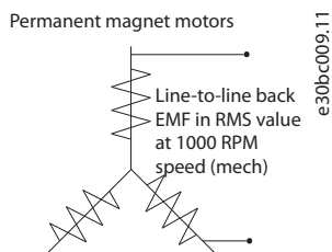
Рисунок 3.7 Определения параметров противо-ЭДС для двигателей с постоянными магнитами
