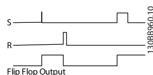
Рисунок 3.43 Выходы триггеров
