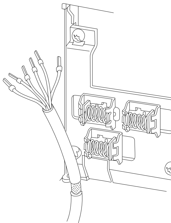
Рисунок 1.5 Заземление экранированных/защищенных кабелей управления
