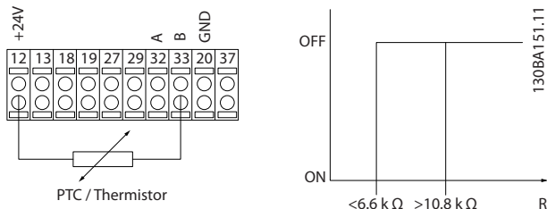
Рисунок 3.16 Подключение термистора
