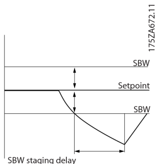
Рисунок 3.97 Задержка выключения насоса (таймер)
